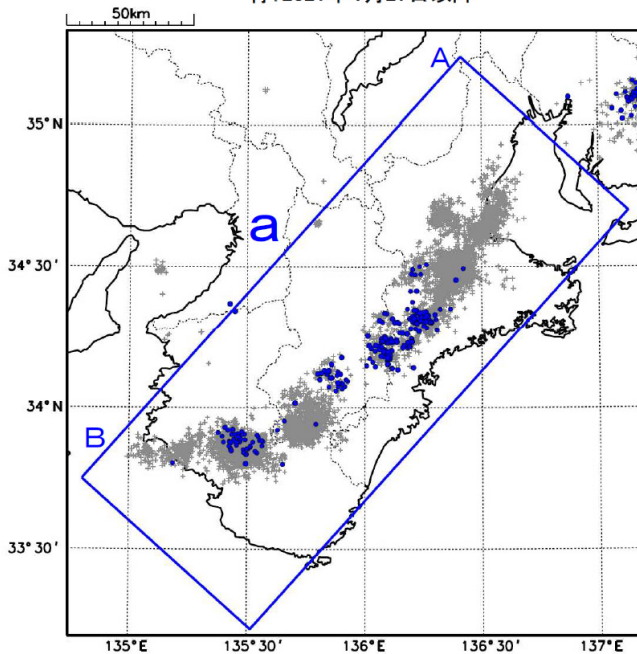
震央分布図（2018年4月1日～2021年5月6日、 深さ0～60km、Mすべて） 灰：2018年4月1日～2021年4月26日、 青：2021年4月27日以降
