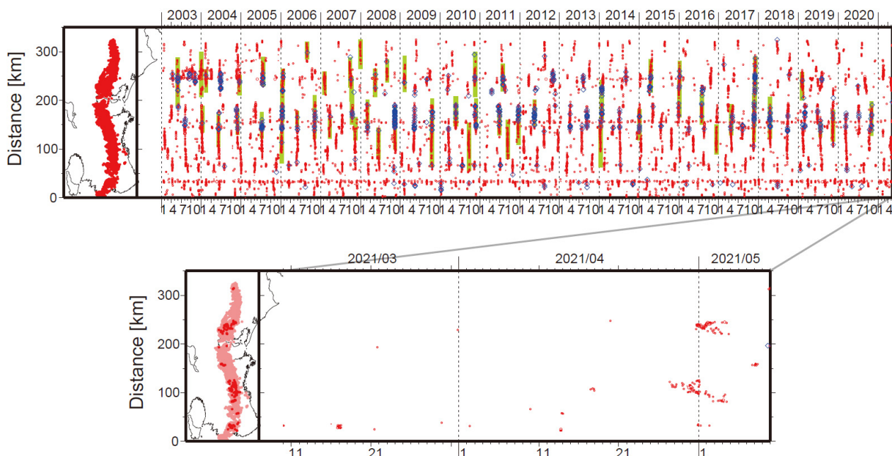
図1. 紀伊半島・東海地域における2003年1月～2021年5月9日までの深部低周波微動の時空間分布（上図）。赤丸はエンベロープ相関・振幅ハイブリッド法 (Maeda and Obara, 2009) およびクラスタ処理 (Obara et al., 2010) によって1時間毎に自動処理された微動分布の重心である。青菱形は周期20秒に卓越する超低周波地震 (Ito et al., 2007) である。黄緑色の太線はこれまでに検出された短期的スロースリップイベント (SSE) を示す。下図は2021年4月を中心とした期間の拡大図である。4月27日～5月4日頃に三重・奈良県境付近から奈良県南部において活発な微動活動がみられた。この活動は三重・奈良県境付近で発生し、南西方向への活動域の移動がみられた。4月30日～5月4日頃には、愛知県西部から中部においてやや活発な活動がみられた。この活動は愛知県西部で開始し、東西両方向に活動域の拡大がややみられた。4月13～14日頃には和歌山県中部から和歌山・奈良県境付近において、4月17日頃には奈良・三重県境付近において、4月30日～5月1日頃には和歌山県中部において、5月7～8日頃には三重県北部において、それぞれごく小規模な活動がみられた。
