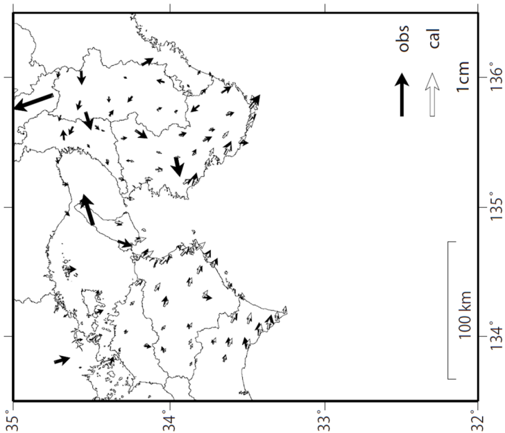
観測値（黒）と計算値（白）の比較 (2020/6/1 - 2021/3/10)
