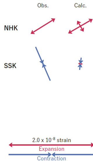
図3 2021/04/09 - 11AM の歪・傾斜変化 (図2[A]) を説明する断層モデル。
