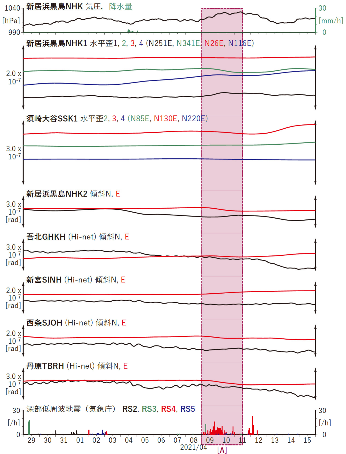
図2 歪・傾斜の時間変化 (2021/03/29 00:00 - 2021/04/16 00:00 (JST))
