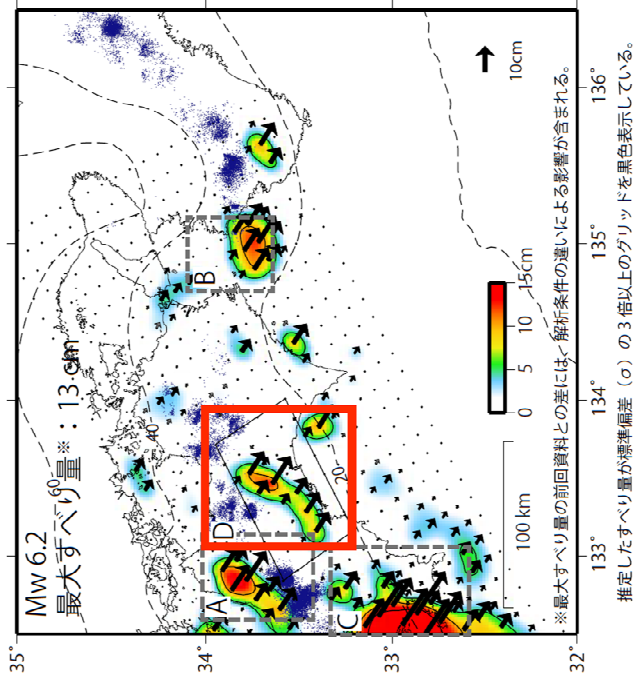
推定すべり分布 (2019/1/1 - 2021/4/8)
