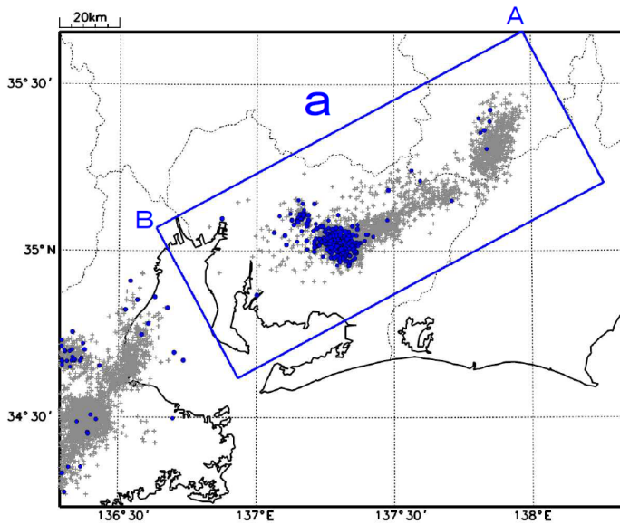
震央分布図（2018年4月1日～2021年5月10日、 深さ0～60km、Mすべて） 灰：2018年4月1日～2021年4月28日、 青：2021年4月29日以降
