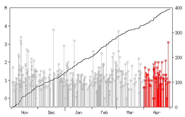
領域d内(日向灘)
