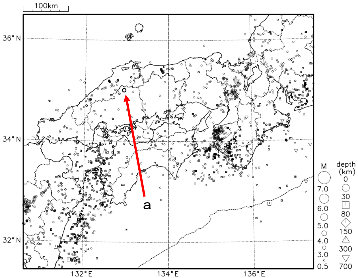
図8 近畿・中国・四国地方の震央分布図（2021年4月1日～4月30日、 M \geq 0.5 ）
