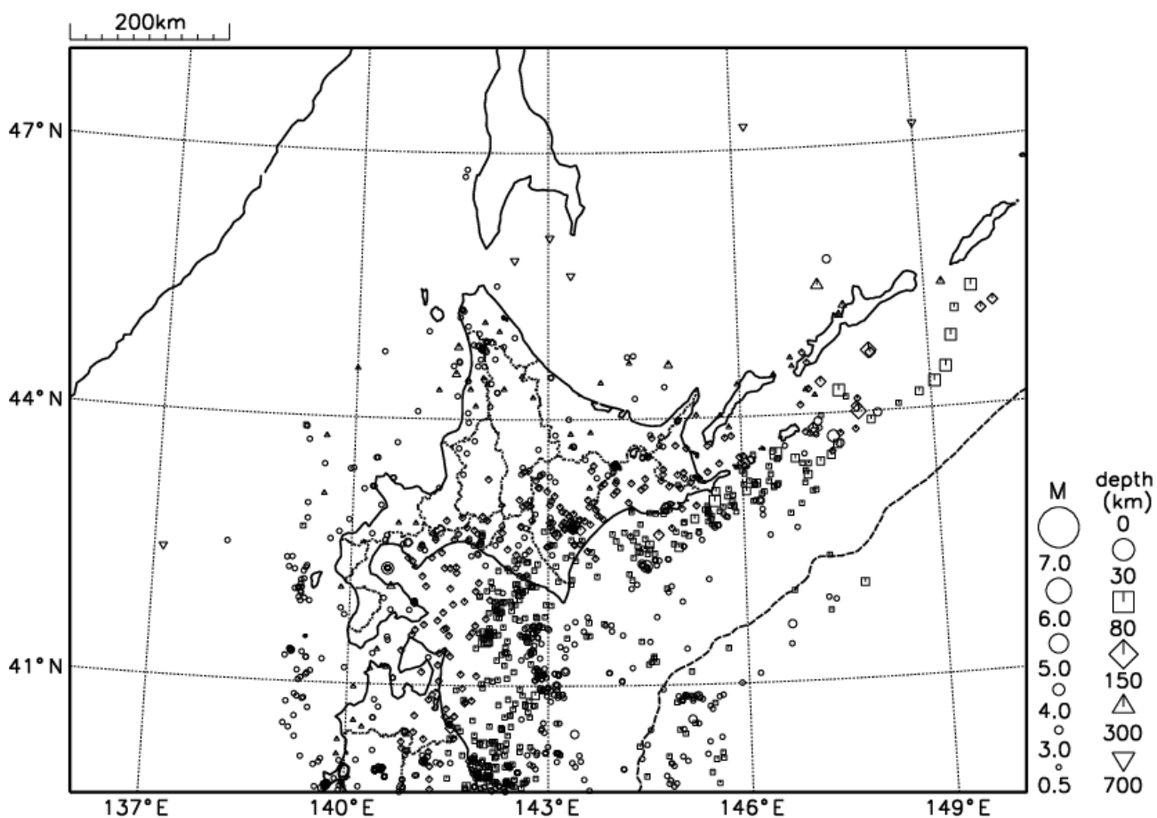
図5 北海道地方の震央分布図（2021年4月1日～4月30日、 M \geq 0.5 ）
