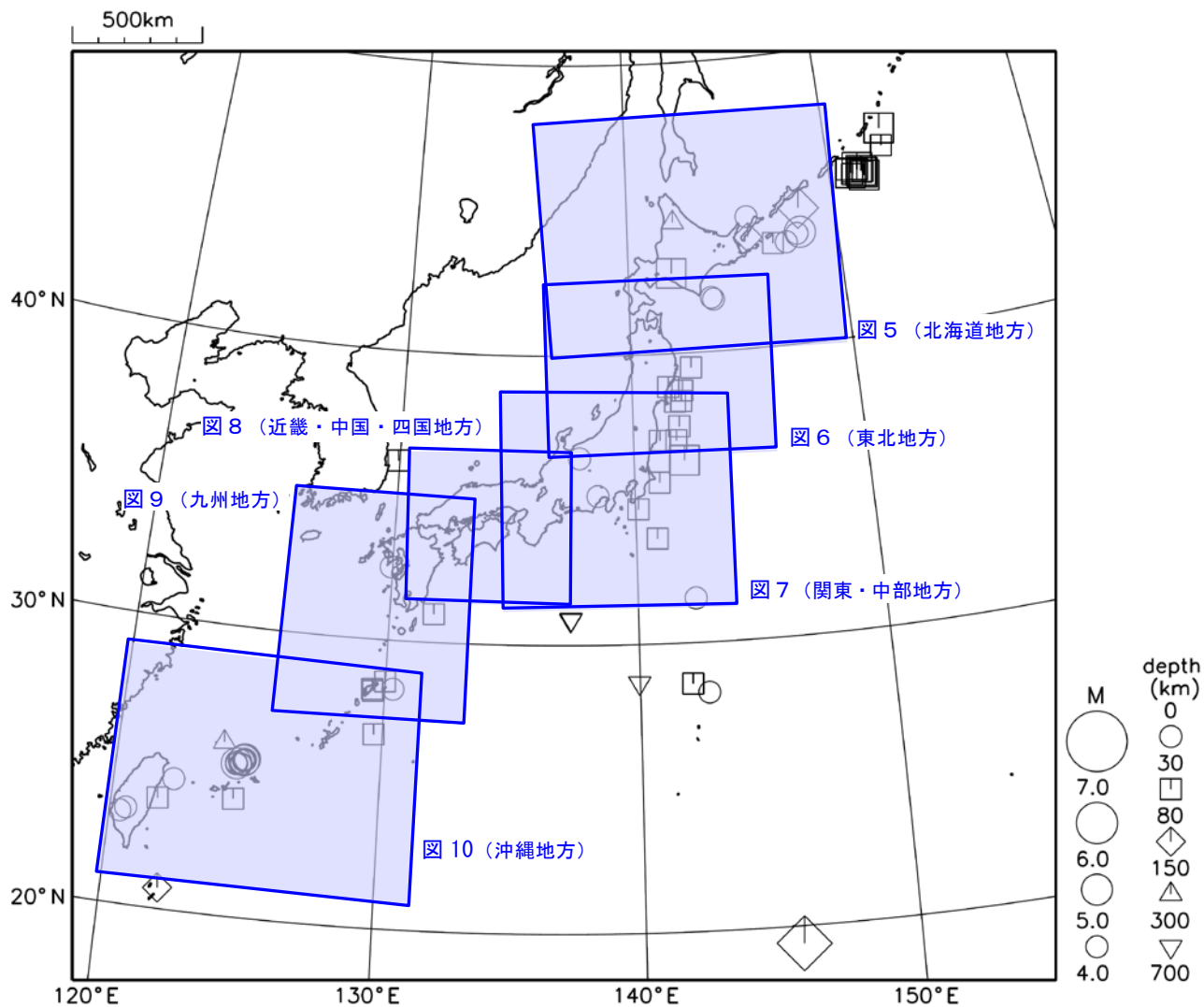
図11 日本周辺で発生した主な地震の震央分布図 (2019年2月1日～2月28日、 M \geq 4.0 )
