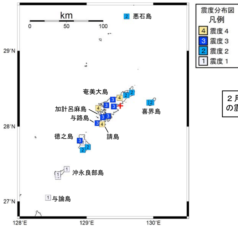
図4 震度分布図
