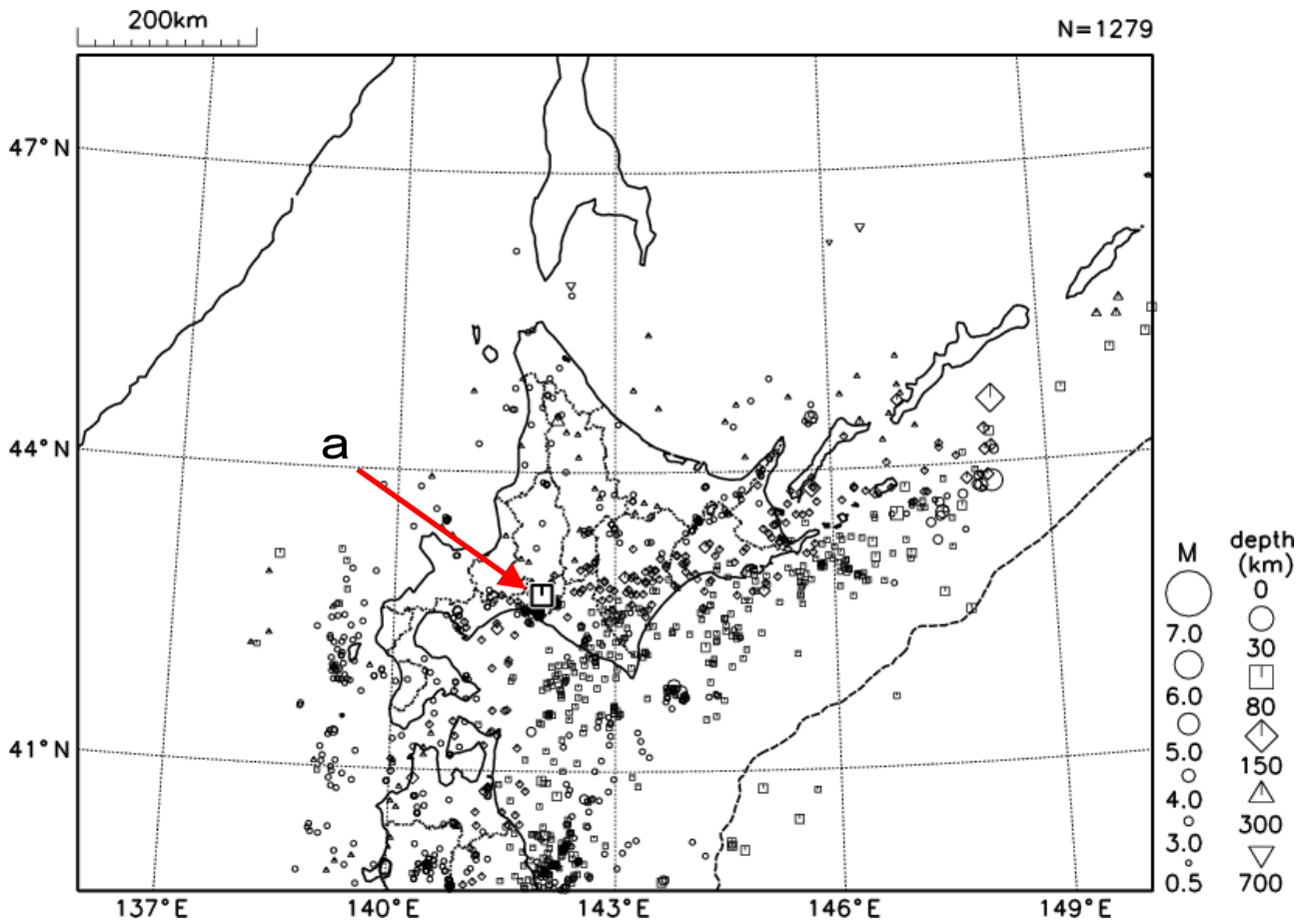
図5 北海道地方の震央分布図 (2019年2月1日～2月28日、 M \geq 0.5 )
