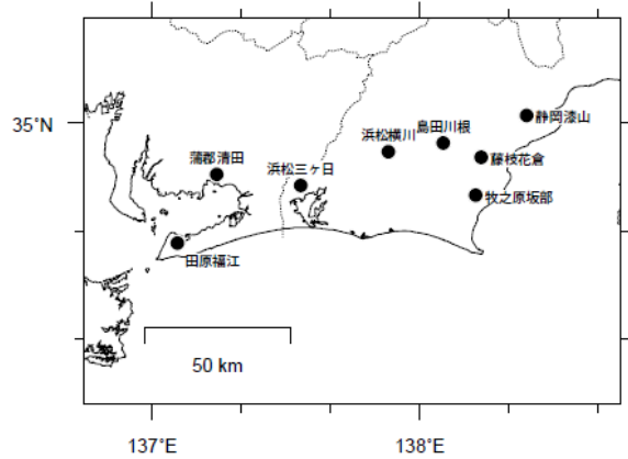
図 3-2 体積ひずみ計の配置図
