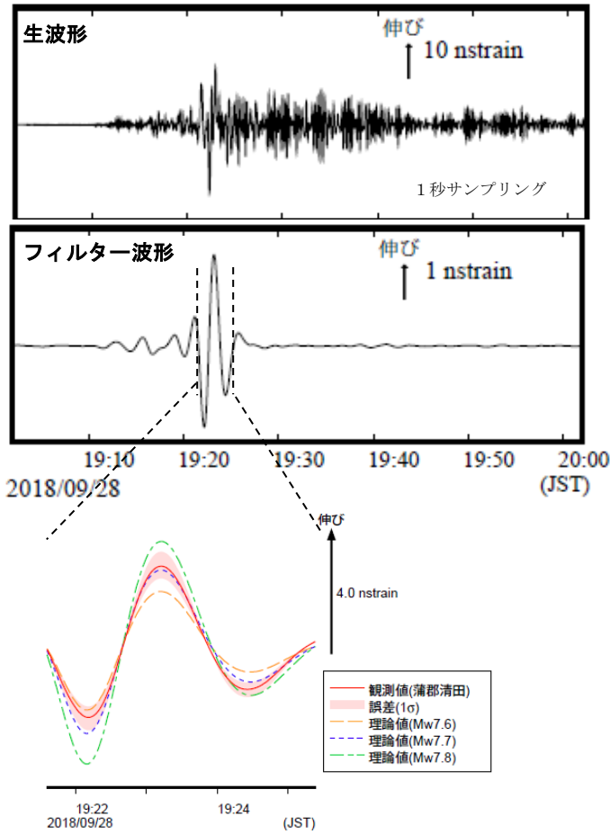
蒲郡清田観測点で観測された体積ひずみ波形
