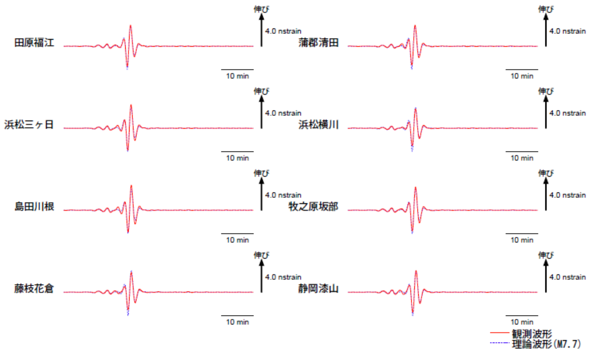
図 3-2 理論波形と体積ひずみ観測点 8 ヲ所の観測波形との比較
