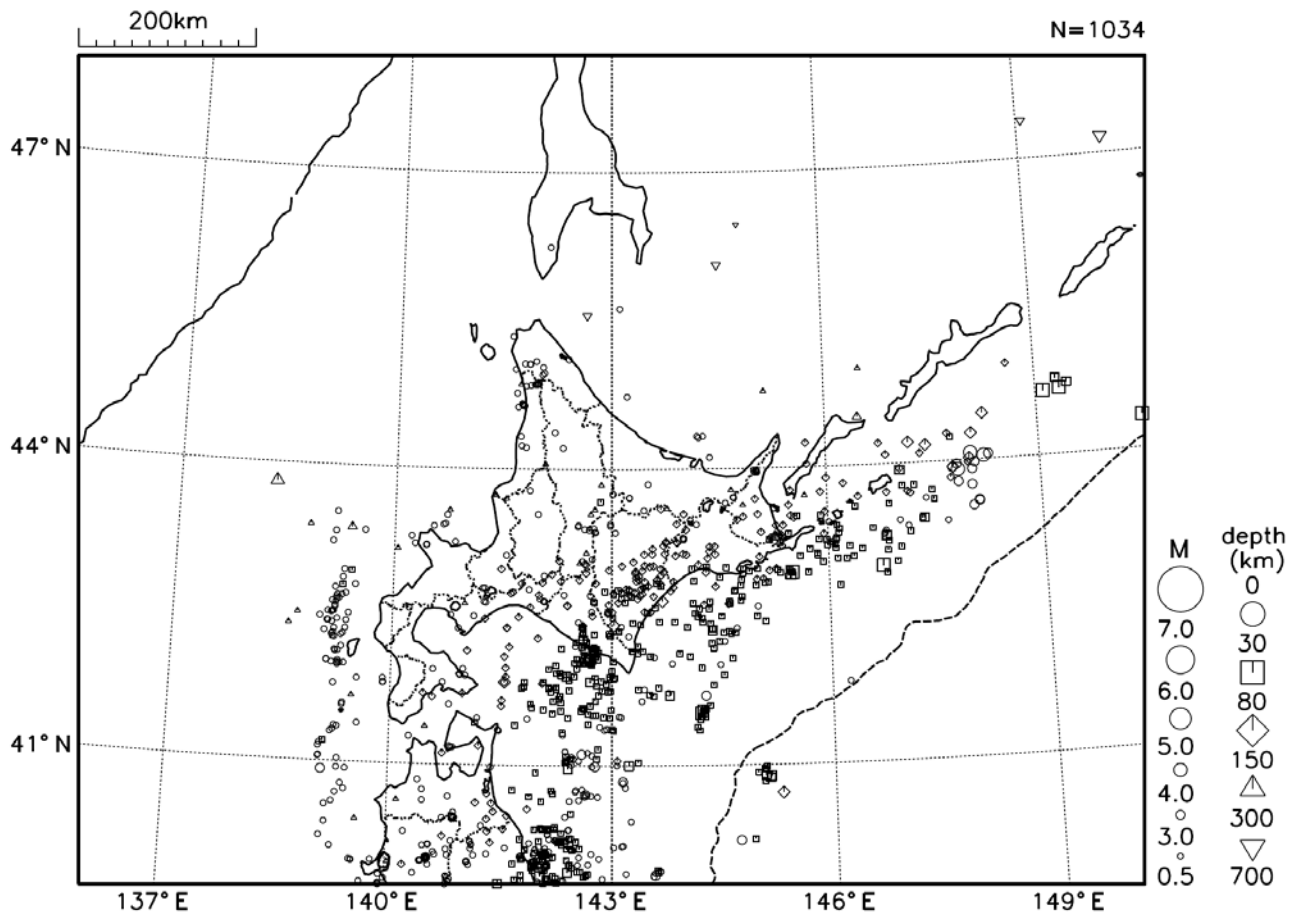
図5 北海道地方の震央分布図 (2018年2月1日～2月28日、 M \geq 0.5 )
