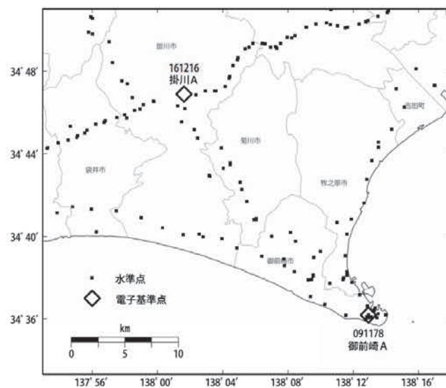
図 9 国土地理院 GNSS 観測結果及び水準測量による御前崎の上下変動
