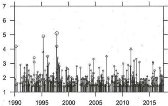
M-I-T図
