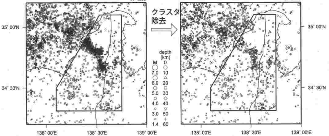
震央分布図
