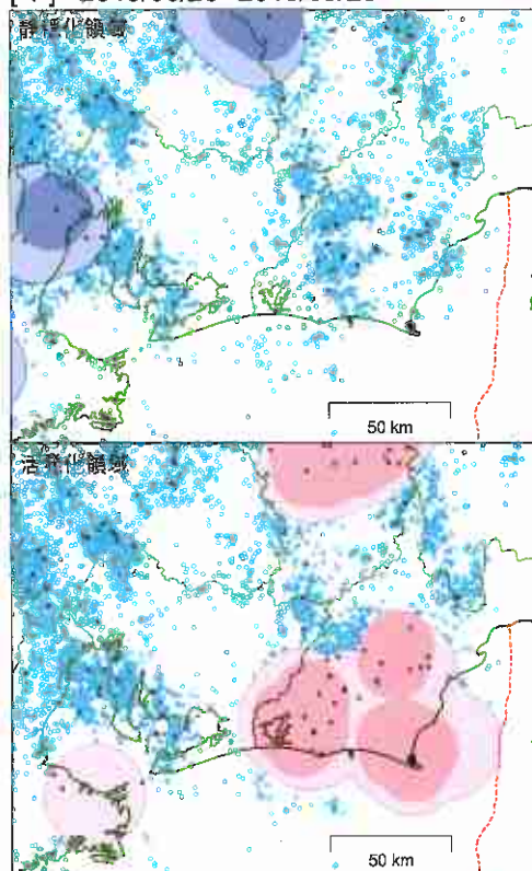
[1] 2015/06/28--2015/09/25
