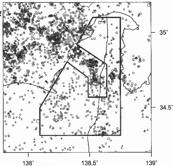
震央分布図
