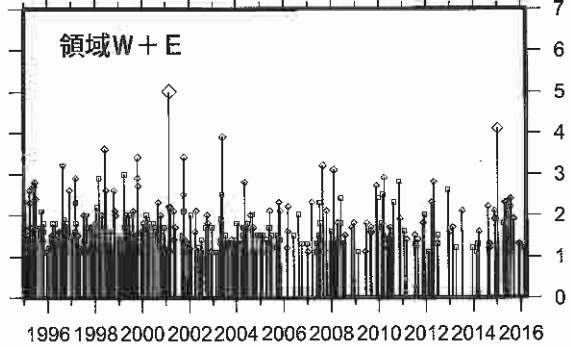
M-T図
