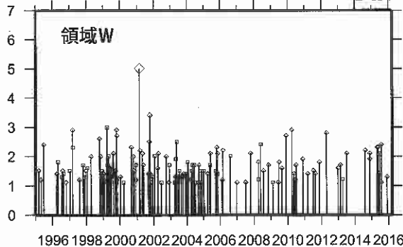
領域W
