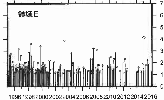
領域E
