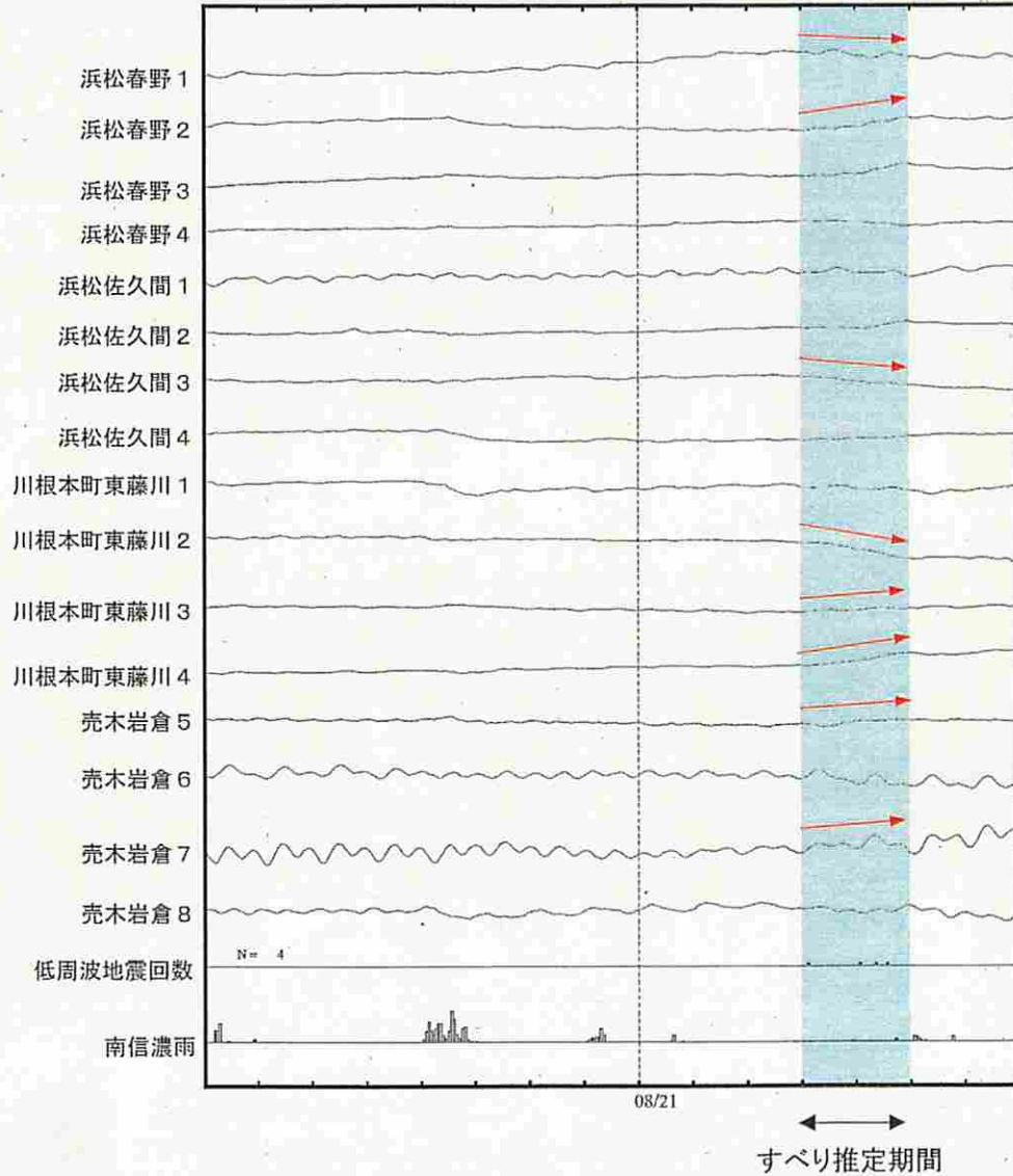
東海周辺ひずみ変化
