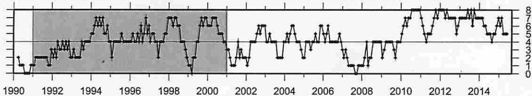
④ 駿河湾（対象期間：180日） 1990/1/1~2015/8/26 M ≥ 1.4
