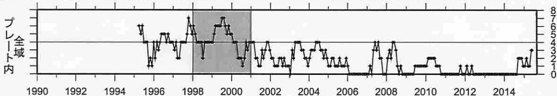
④ 駿河湾（対象期間：180日） 1990/1/1~2015/8/26 M ≥ 1.4
