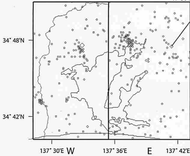
震央分布図
