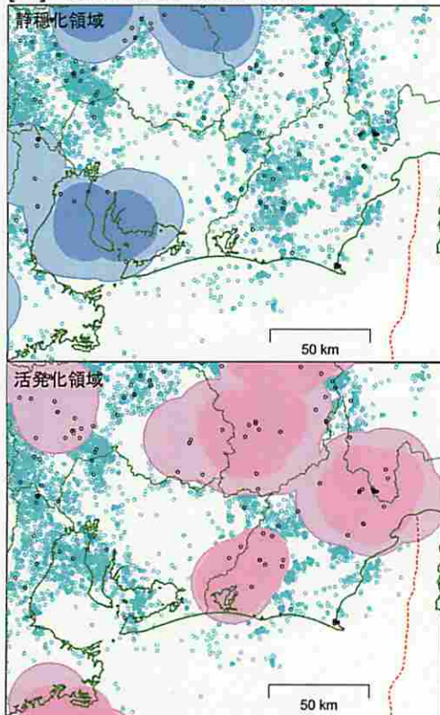
[ 2 ] 2014/07/26--2014/10/23
