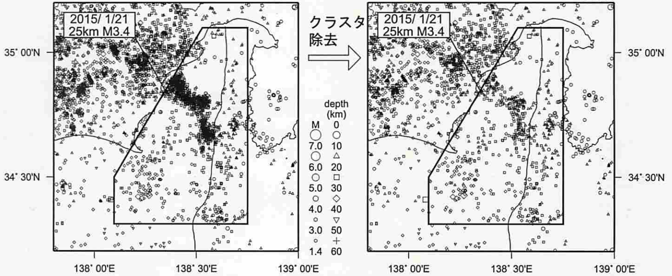
震央分布図
