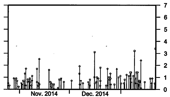
M-I図
