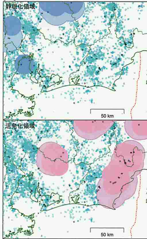
[ 1 ] 2014/04/27--2014/07/25
