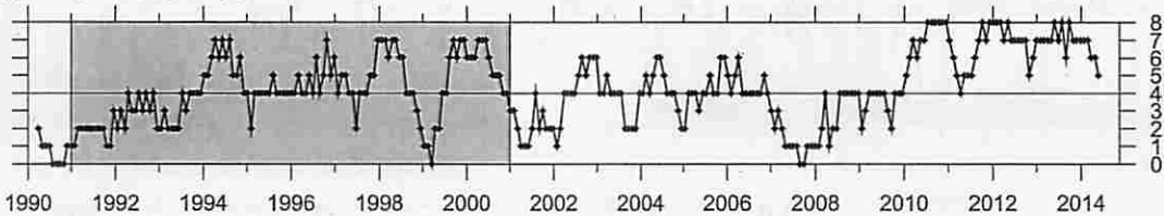
④ 駿河湾（対象期間：180日） 1990/1/1~2014/11/13 M ≥ 1.4
