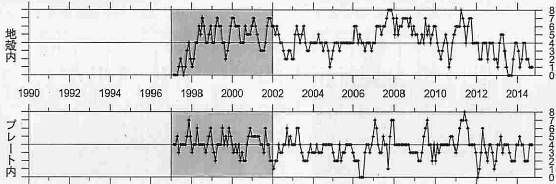
② 愛知県（対象期間：90日） 1997/1/1~2014/11/13 M ≥ 1.1
