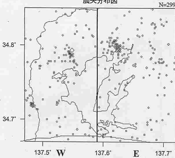
震央分布図
