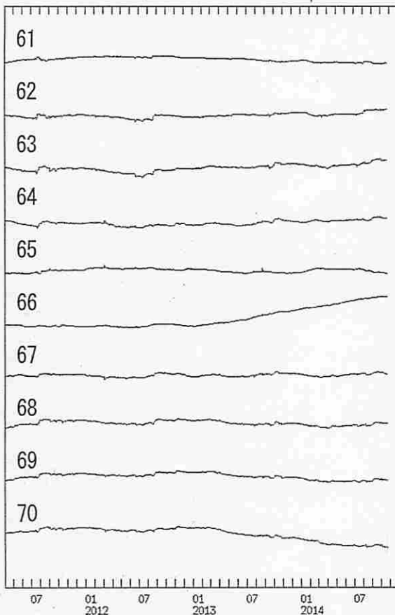
図1：日値スタッキング波形。番号は監視グリッド（図2参照）を示す。
