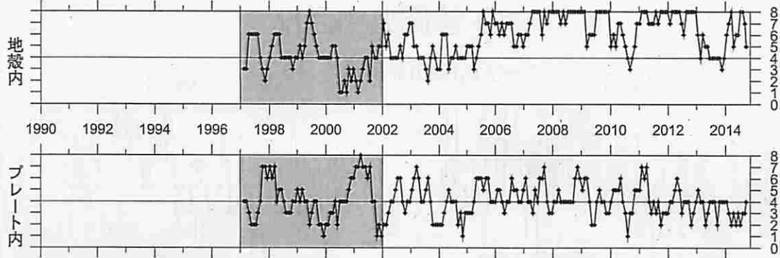
① 静岡県中西部（対象期間：90日） 1997/1/1~2014/11/13 M ≥ 1.1
