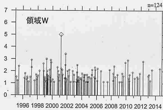
M-T図
