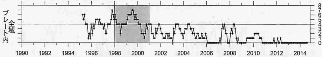
④ 駿河湾（対象期間：180日） 1990/1/1~2014/11/13 M ≥ 1.4
