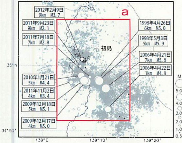
震央分布図（1997年10月1日～2012年3月21日、 M \geq 0.5 、深さ0～20km）
