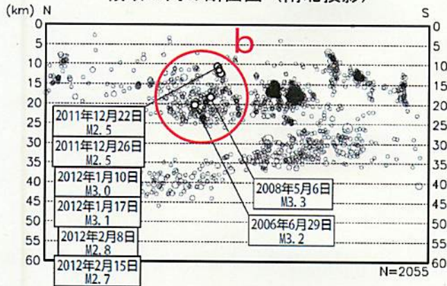
領域a内の断面図 (南北投影)
