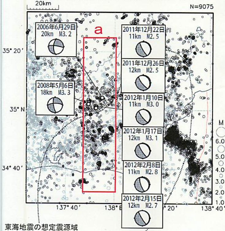
震央分布図 (1997年10月1日~2012年3月21日、 M \geq 1.0 、深さ0~60km)
