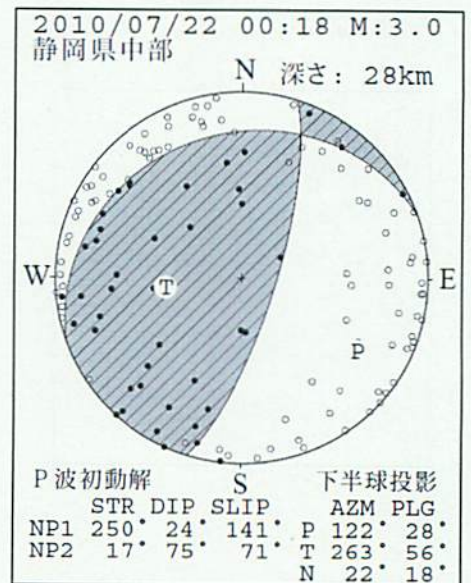
今回の地震の発震機構及びその断層パラメータ
