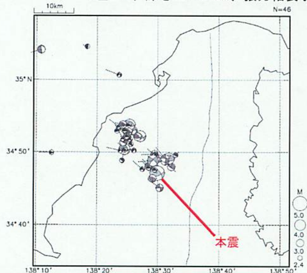
発震機構の分布図 (2009年8月11日~2010年7月21日、 M \geq 2.4 、深さ25~60km、張力軸表示)
