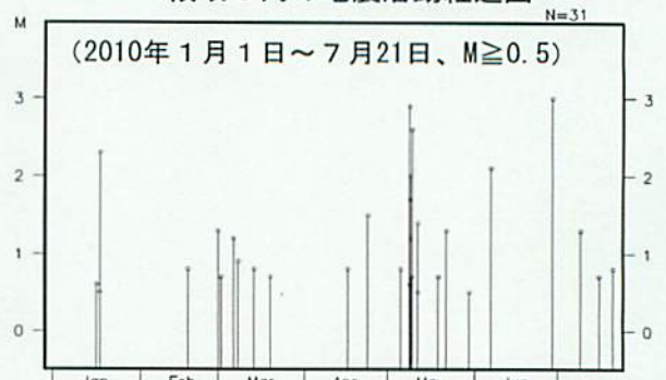
領域c内の地震活動経過図
