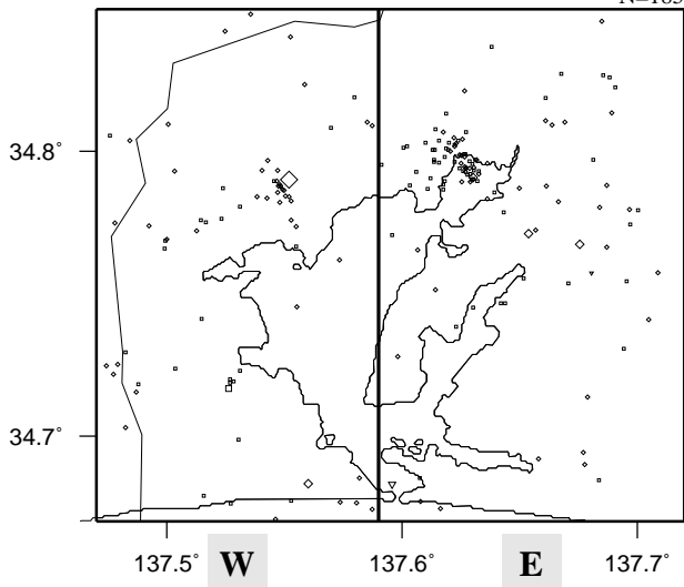
震央分布図
