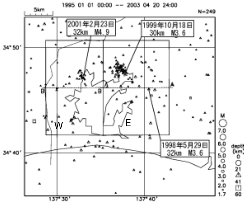
震央分布図
