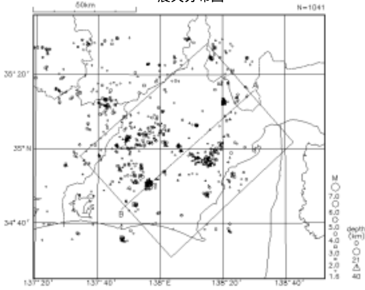
震央分布図
