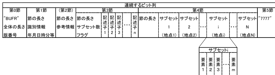
図 1－1 BUFR 報の構成
