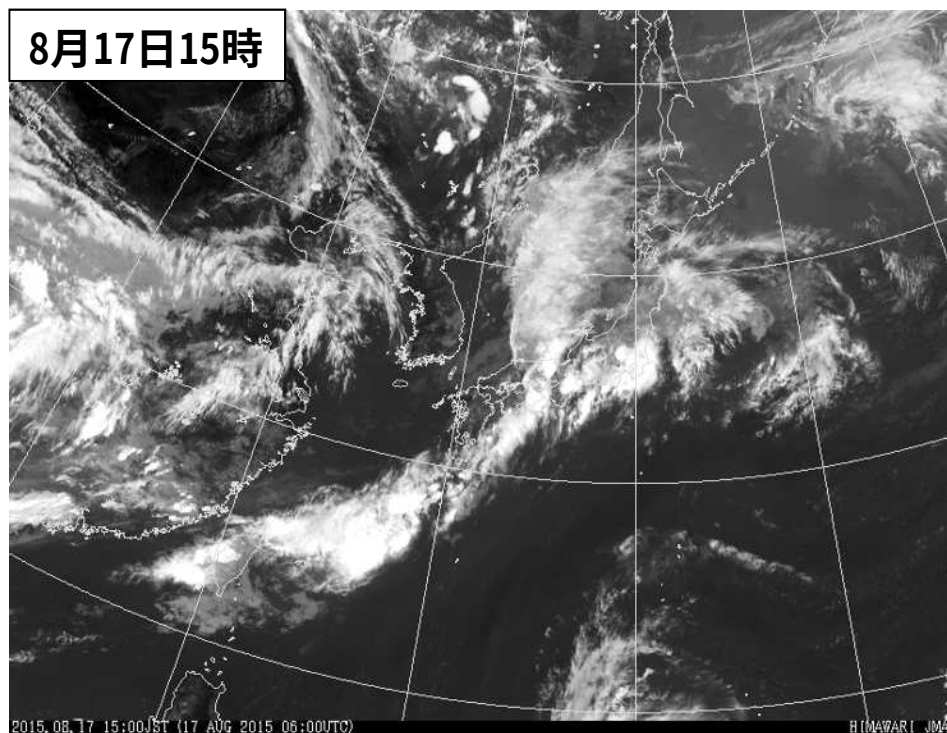
地上天気図および気象衛星「ひまわり8号」赤外画像 平成27年8月17日15時
