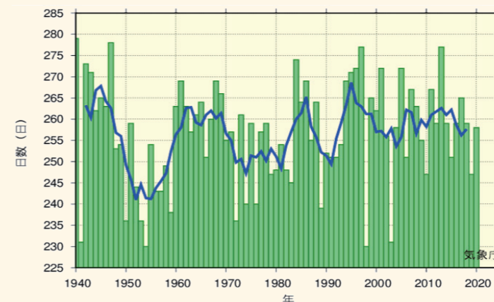
静岡(静岡市)の年間無降水日数
