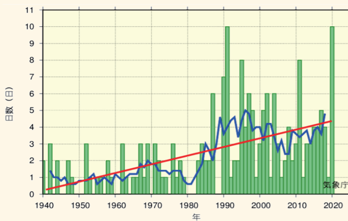
静岡(静岡市)の年間猛暑日日数
