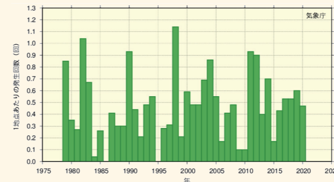
静岡県の1時間降水量50mm以上の発生回数変化
