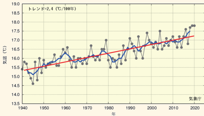
静岡(静岡市)の年平均気温
