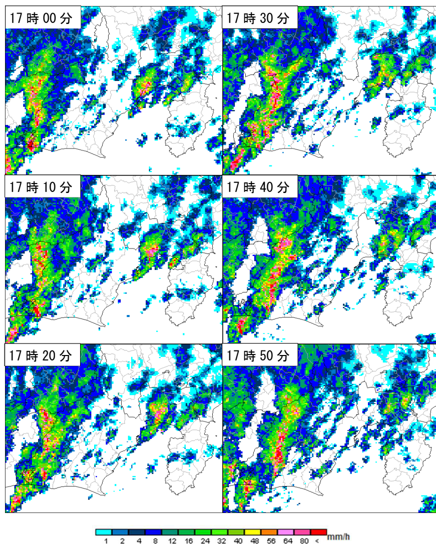
7月26日17時00分から10分毎のレーダー画像
