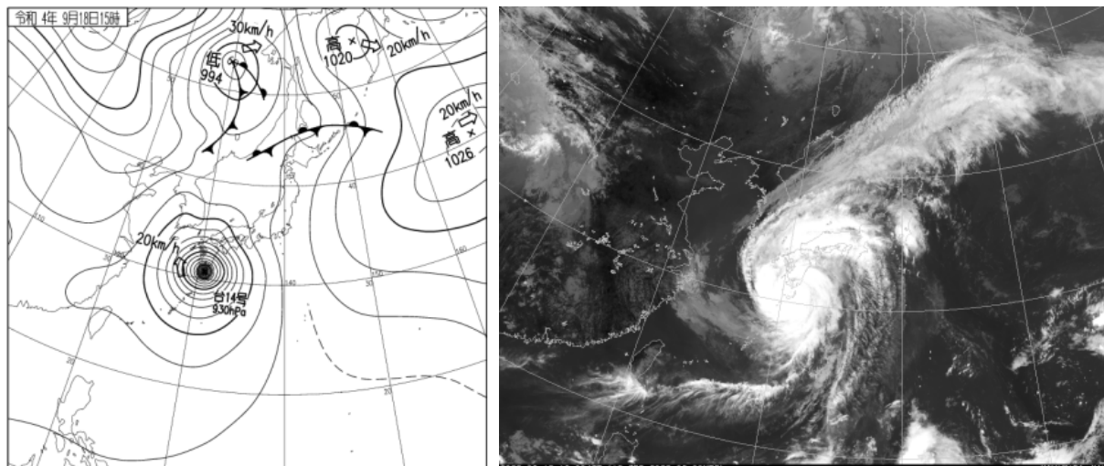
9 月 18 日 15 時の地上天気図（左）と気象衛星赤外画像（右）
