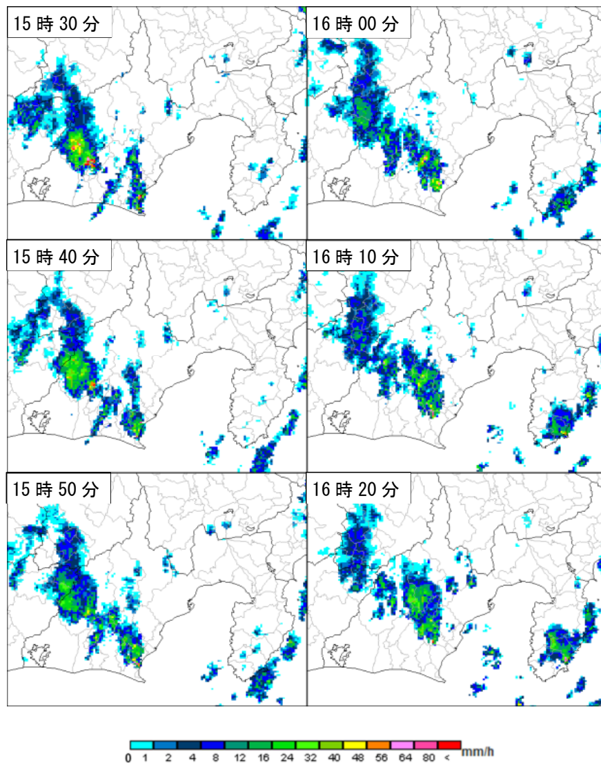
9 月 18 日 15 時 30 分から 10 分毎のレーダー画像
