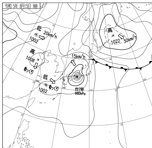
8月15日09時の地上天気図（左）と気象衛星赤外面像（右）
