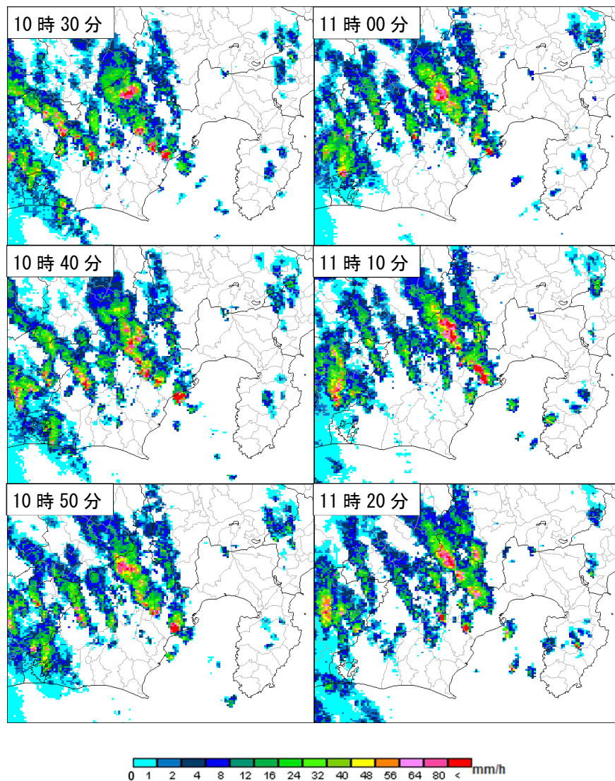
8月15日10時30分から10分毎の気象レーダー画像
