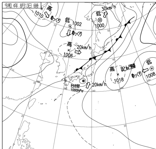
8月13日06時の地上天気図（左）と気象衛星赤外面像（右）
