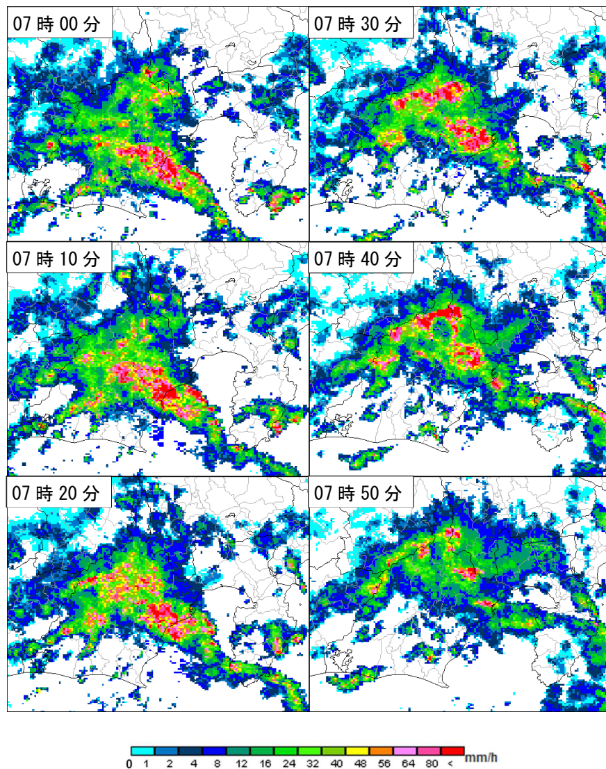
8 月 13 日 07 時 00 分から 10 分毎のレーダー画像
