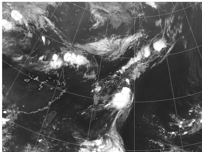
8月13日06時の地上天気図（左）と気象衛星赤外面像（右）
