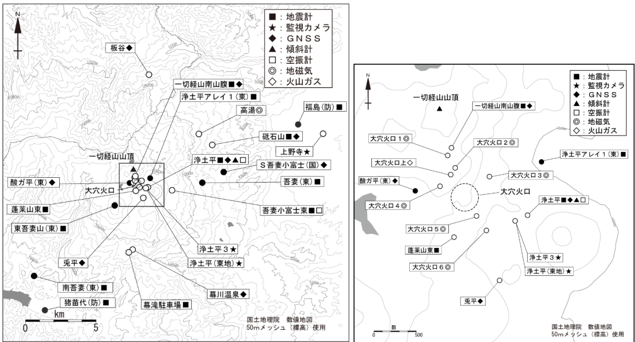
図6 吾妻山 観測点配置図
