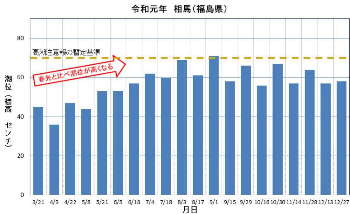
図 1-2 大潮の時期における最高潮位の予測値（相馬（福島県））
