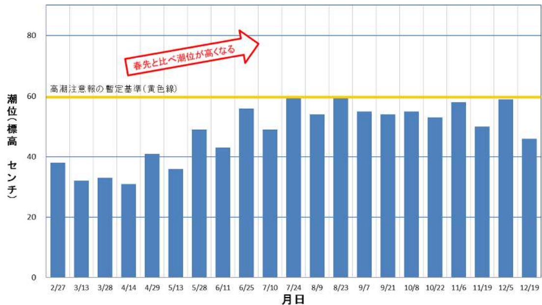
図 1-3 大潮の時期における最高潮位の予測値(相馬(福島県))
