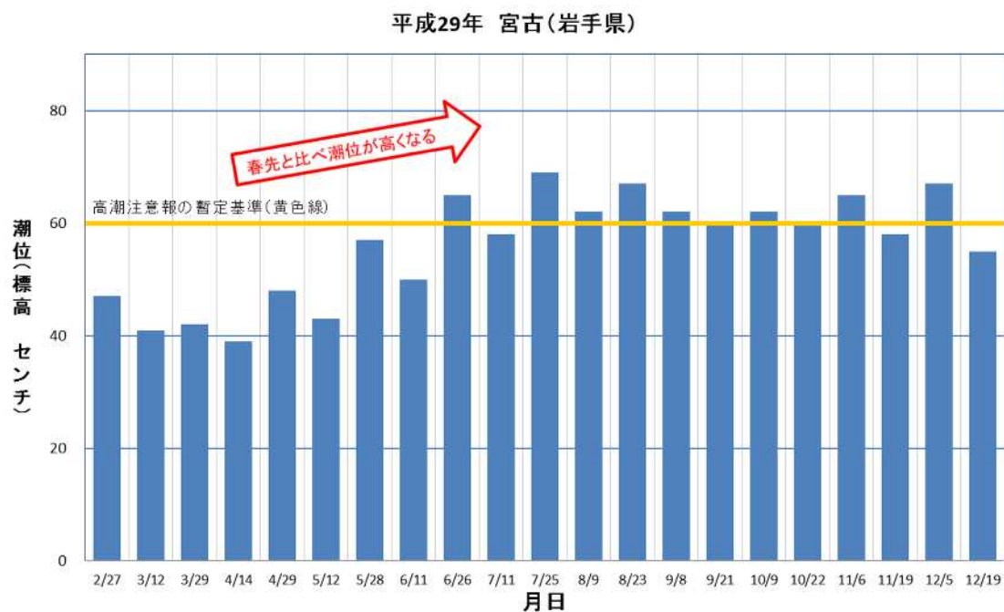
図 1-1 大潮の時期における最高潮位の予測値(宮古(岩手県))
