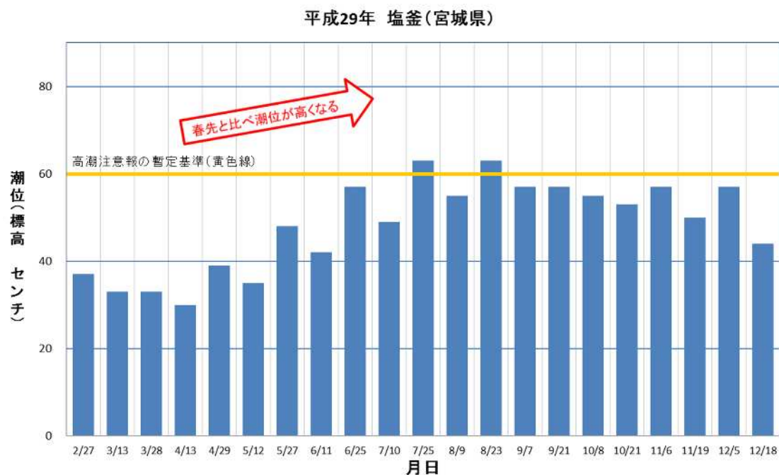
図 1-2 大潮の時期における最高潮位の予測値(塩釜(宮城県))
