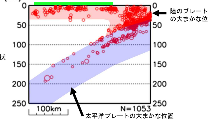
(km) 福島県付近の断面図 (G-H 投影)
