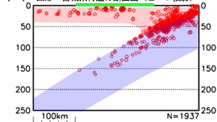
(km) 山形・宮城県付近の断面図 (E-F 投影)
