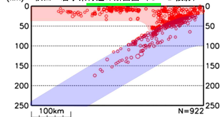
(km) 秋田・岩手県付近の断面図 (C-D 投影)
