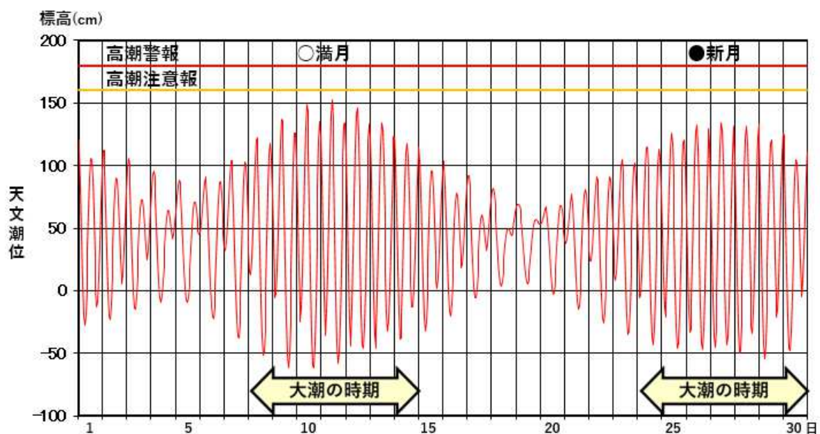
図3 唐津における2022年9月(1時間ごとの)の天文潮位
