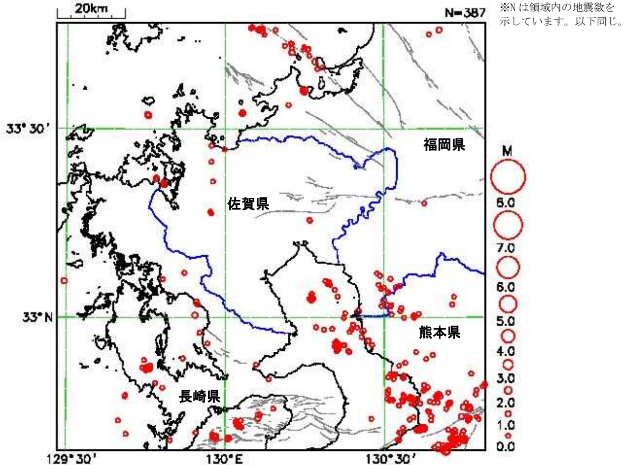
図 1 震央分布図 (2024 年 6 月 1 日～30 日、深さ 30km 以浅、 M \geq 0.0 ) 灰色の線は地震調査研究推進本部の長期評価による活断層を示しています。
