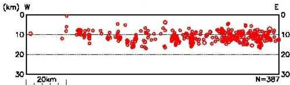
図 2 断面図 (2024 年 6 月 1 日～30 日、深さ 30km 以浅) 震央分布図を南の方から見た断面図です。
