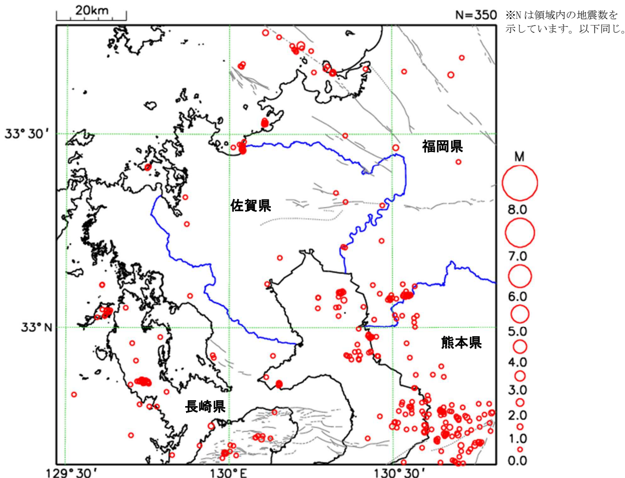
図 1 震央分布図 (2023 年 9 月 1 日~30 日、深さ 30km 以浅、 M \geq 0.0 ) 灰色の線は地震調査研究推進本部の長期評価による活断層を示しています。
