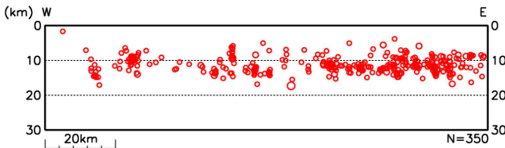
図 2 断面図 (2023 年 9 月 1 日~30 日、深さ 30km 以浅) 震央分布図を南の方から見た断面図です。
