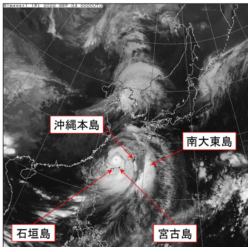
気象衛星画像（赤外）2022年9月4日09時
