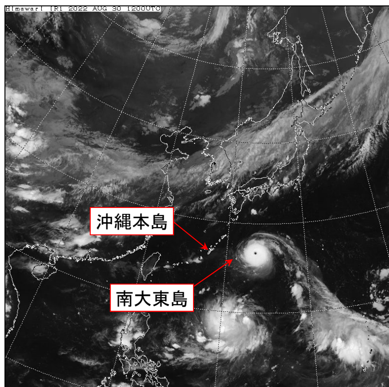
気象衛星画像（赤外）2022年8月30日21時
