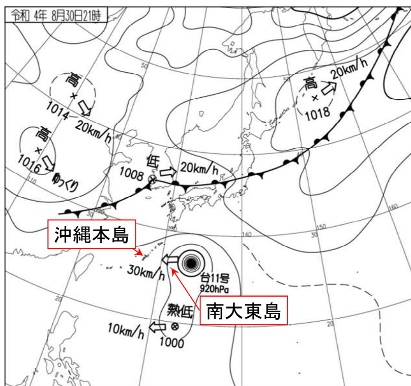
地上天気図 2022年8月30日21時
