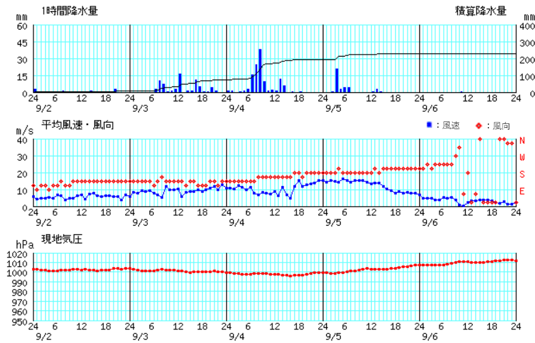
伊是名 2022年9月2日00時～2022年9月6日24時
