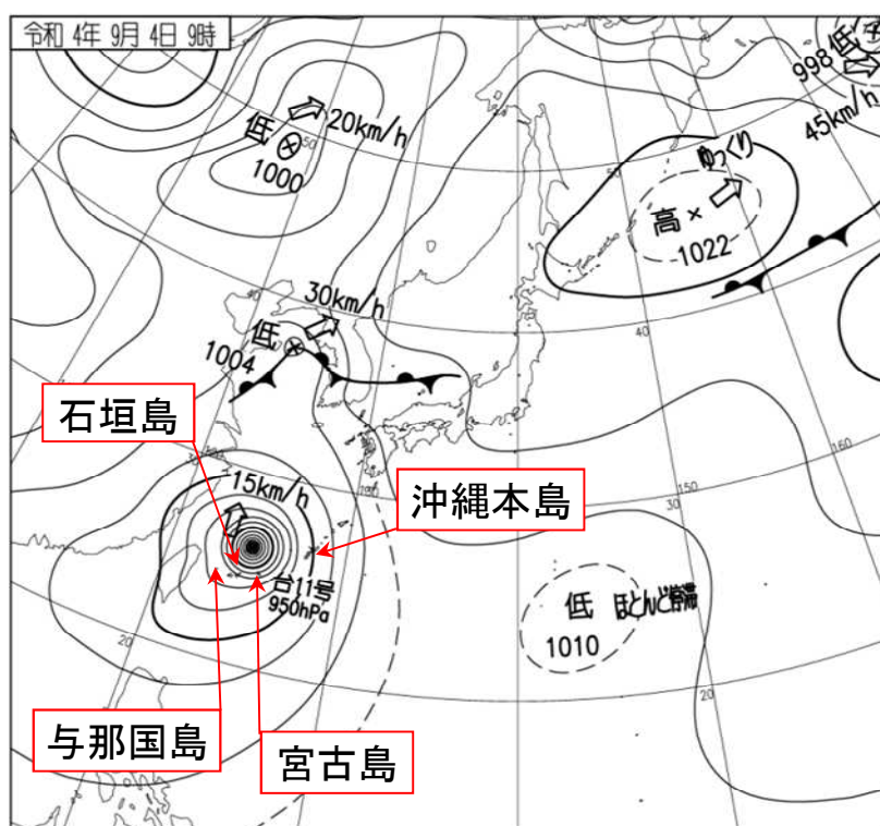
地上天気図 2022年9月4日09時
