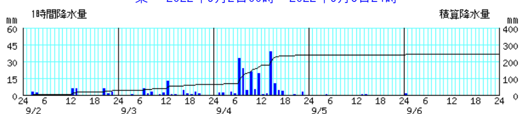
栗国 2022年9月2日00時～2022年9月6日24時
