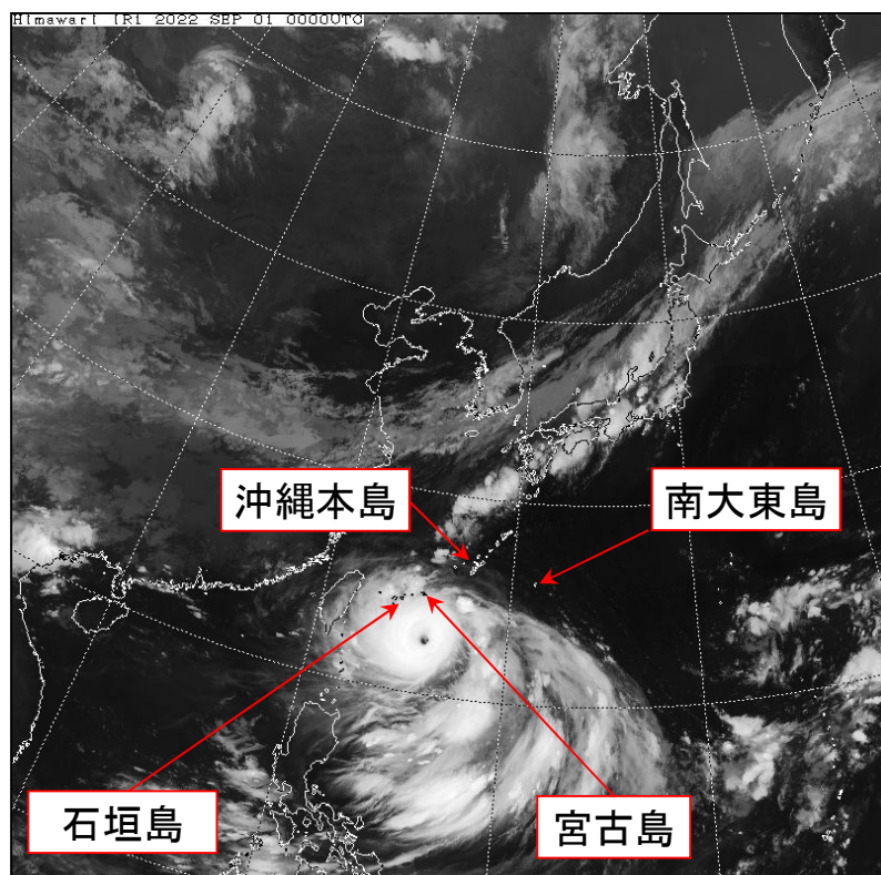
気象衛星画像（赤外）2022年9月1日09時
