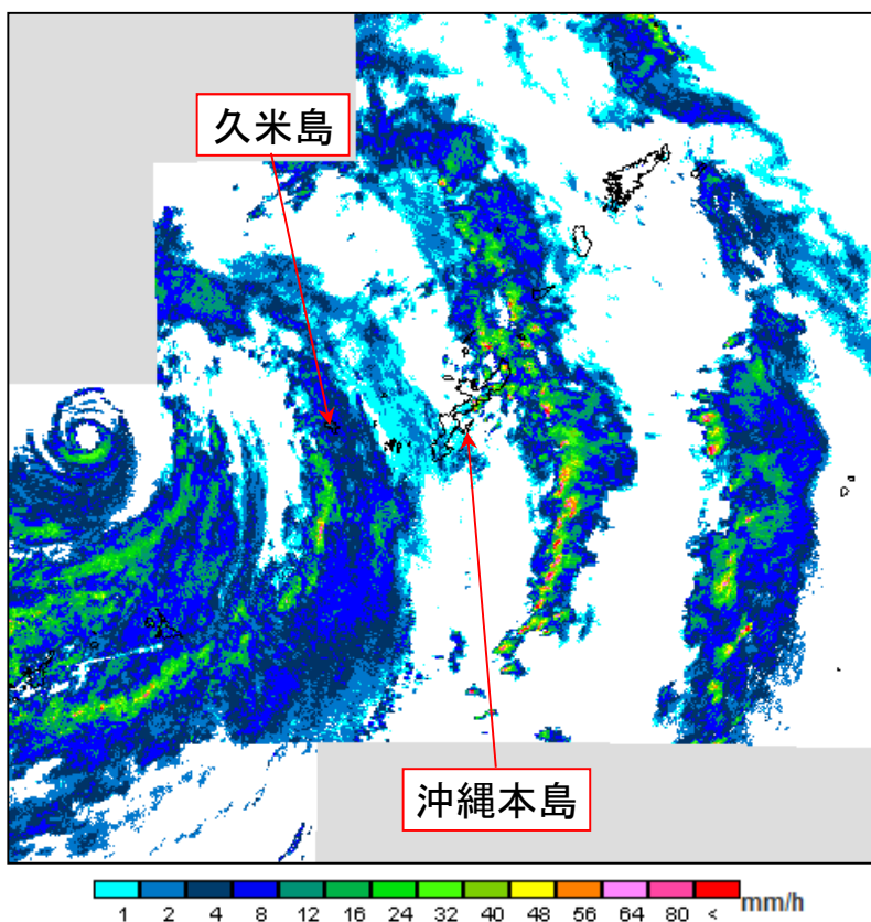
気象レーダー（降水強度）2022年9月4日12時
