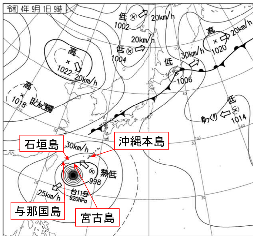
地上天気図 2022年9月1日09時
