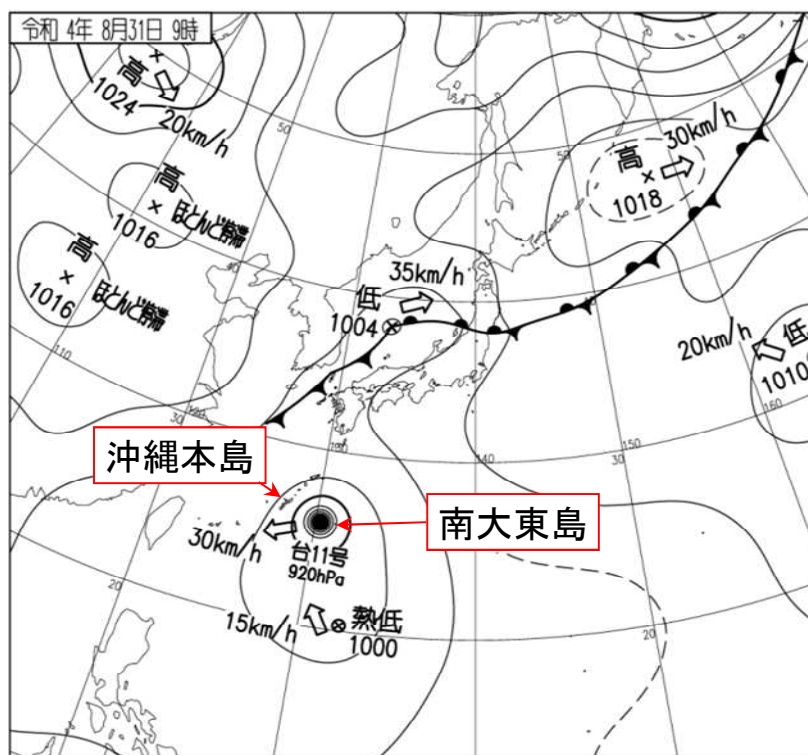
地上天気図 2022年8月31日09時
