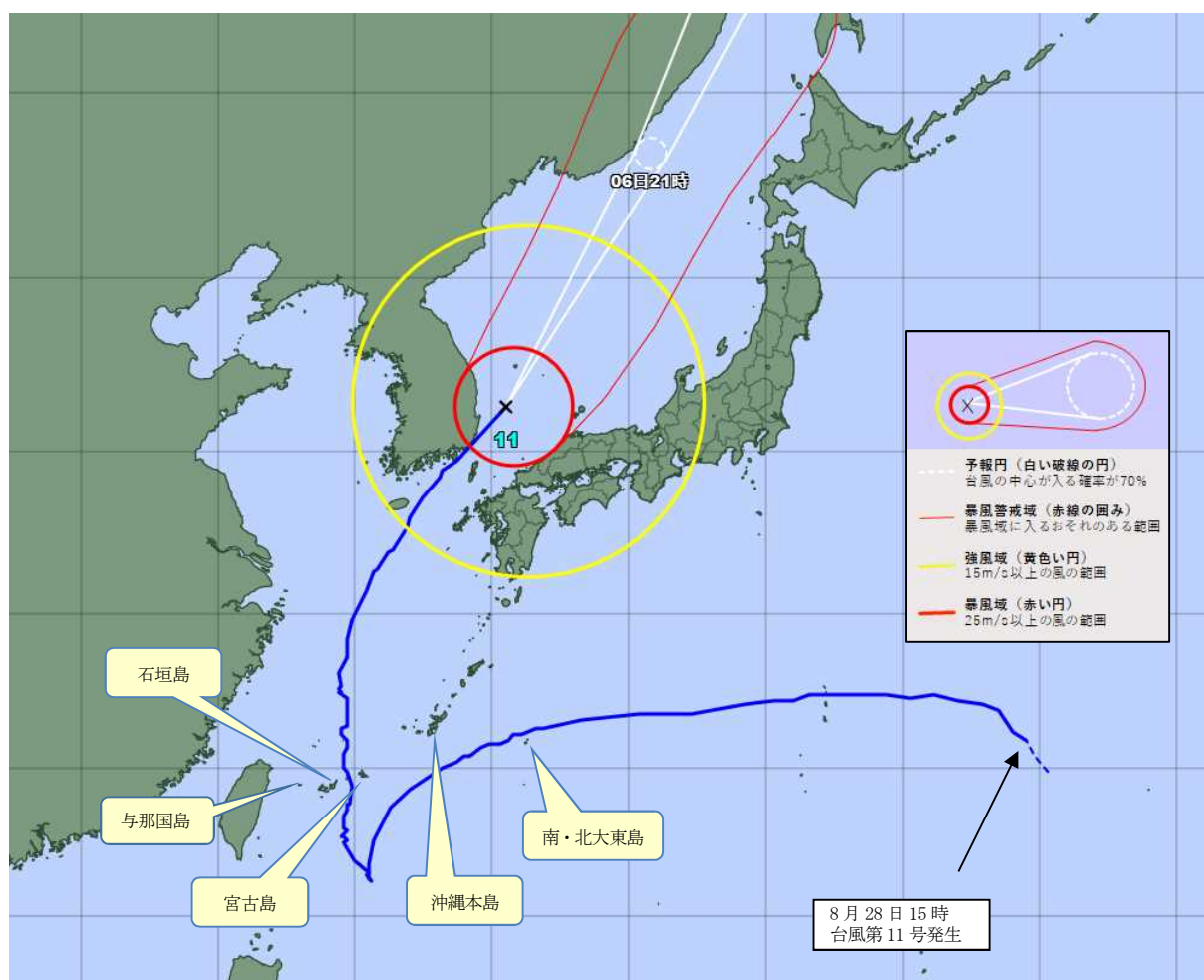
台風第11号経路図（2022年9月6日09時現在 速報値）
