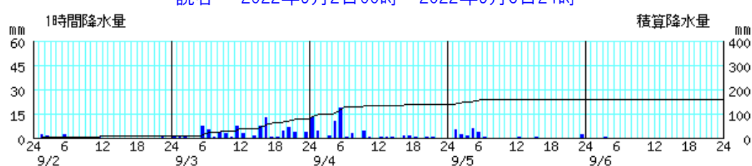
読谷 2022年9月2日00時～2022年9月6日24時
