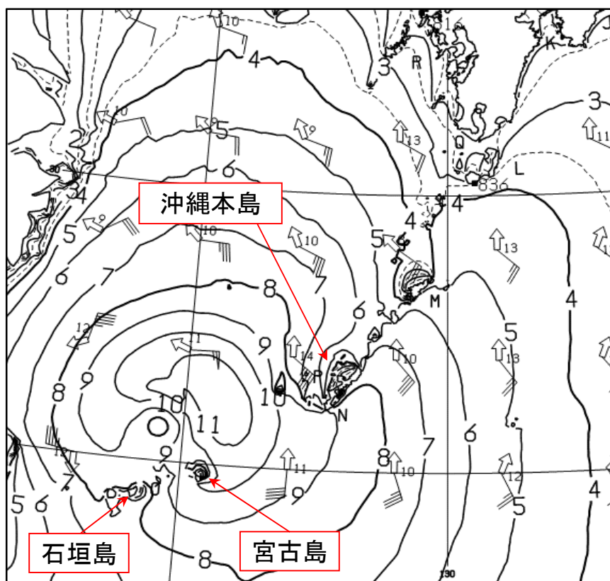
沿岸波浪実況図 2022年9月4日09時
