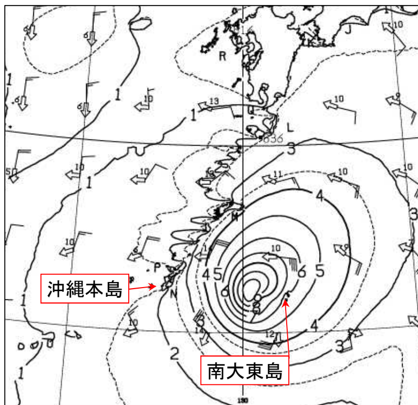
沿岸波浪実況図 2022年8月30日21時
