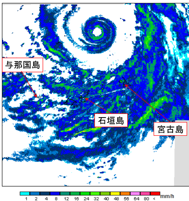
気象レーダー（降水強度）2022年9月4日09時
