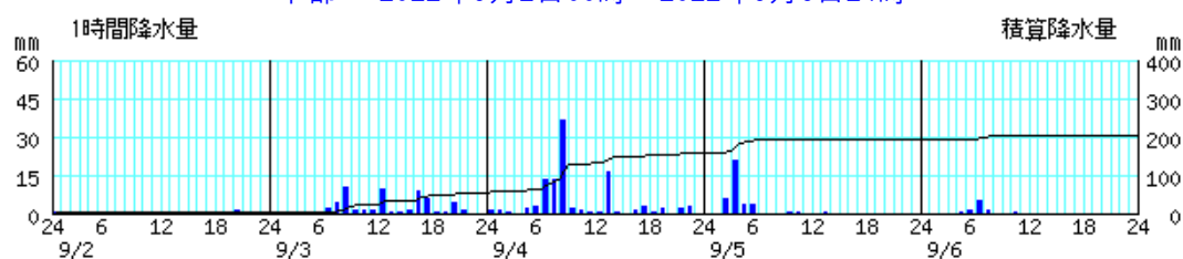
東 2022年9月2日00時～2022年9月6日24時
