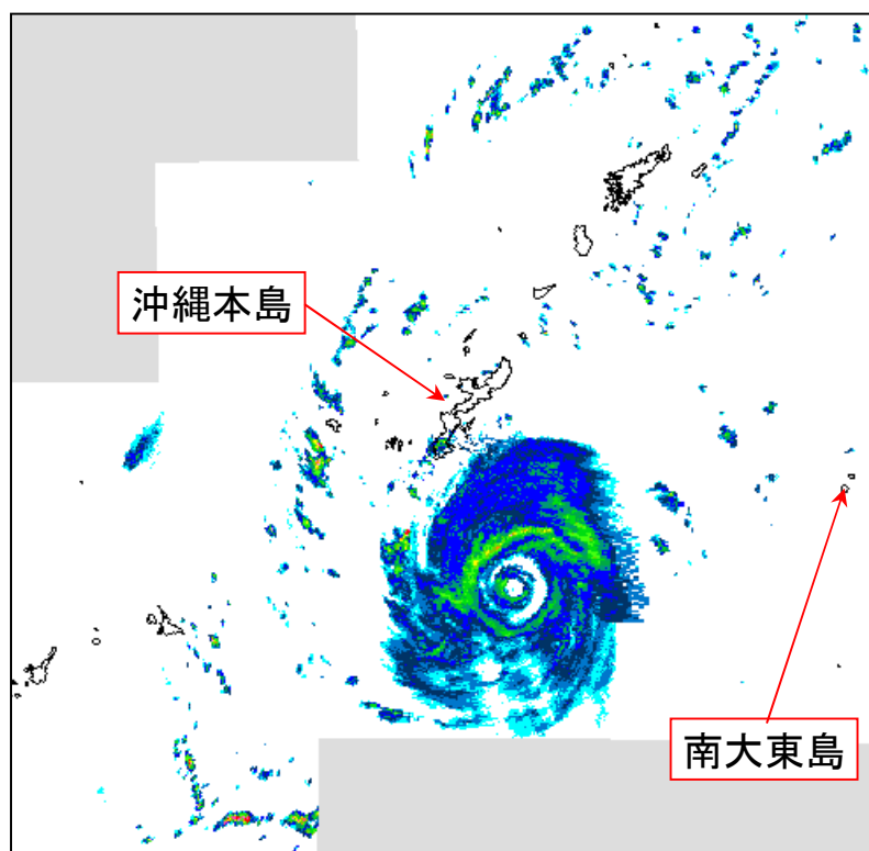
気象レーダー（降水強度）2022年8月31日18時
