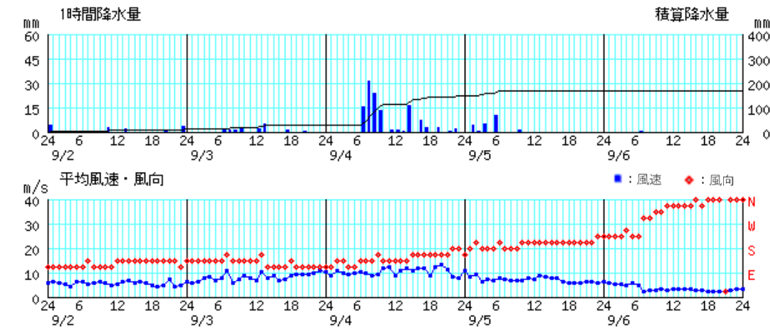
奥 2022年9月2日00時～2022年9月6日24時
