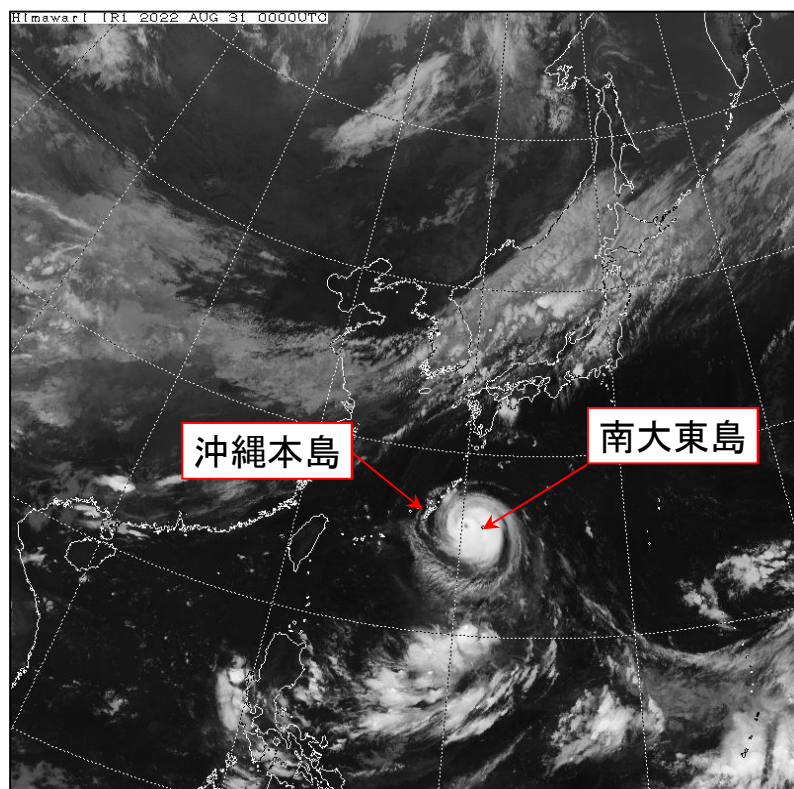
気象衛星画像（赤外）2022年8月31日09時
