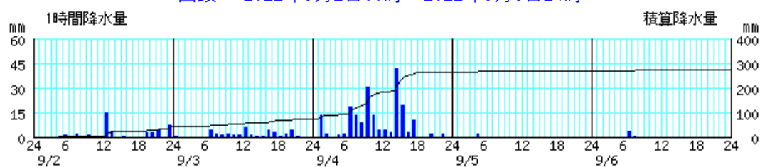
本部 2022年9月2日00時～2022年9月6日24時
