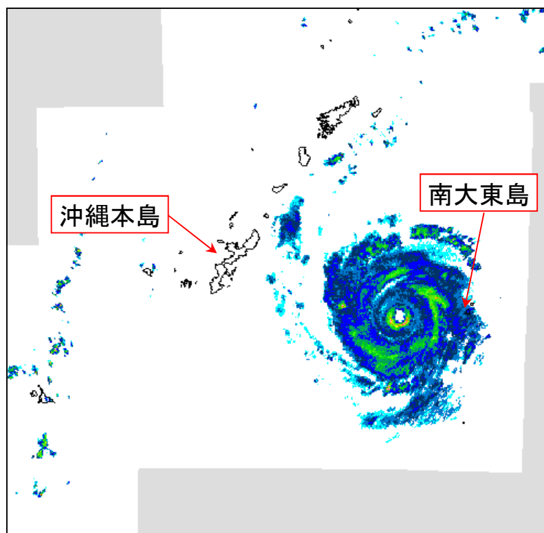
気象レーダー（降水強度）2022年8月31日09時
