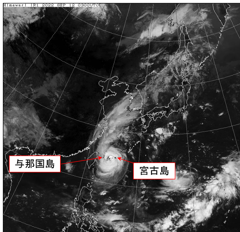
気象衛星画像（赤外） 2022年9月12日12時
