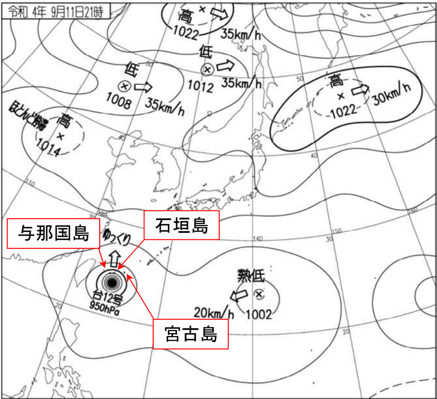
地上天気図 2022年9月11日21時
