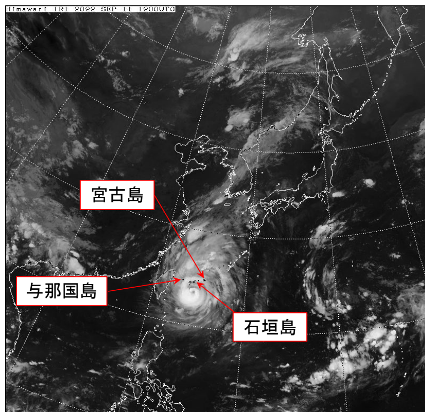
気象衛星画像（赤外） 2022年9月11日21時
