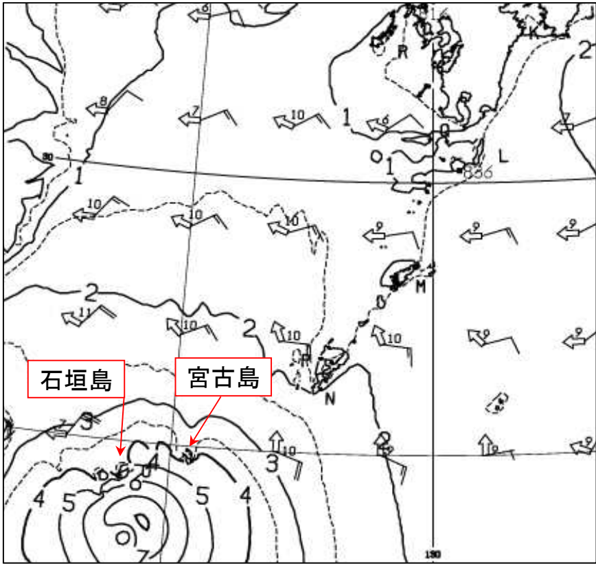
沿岸波浪実況図 2022年9月11日21時
