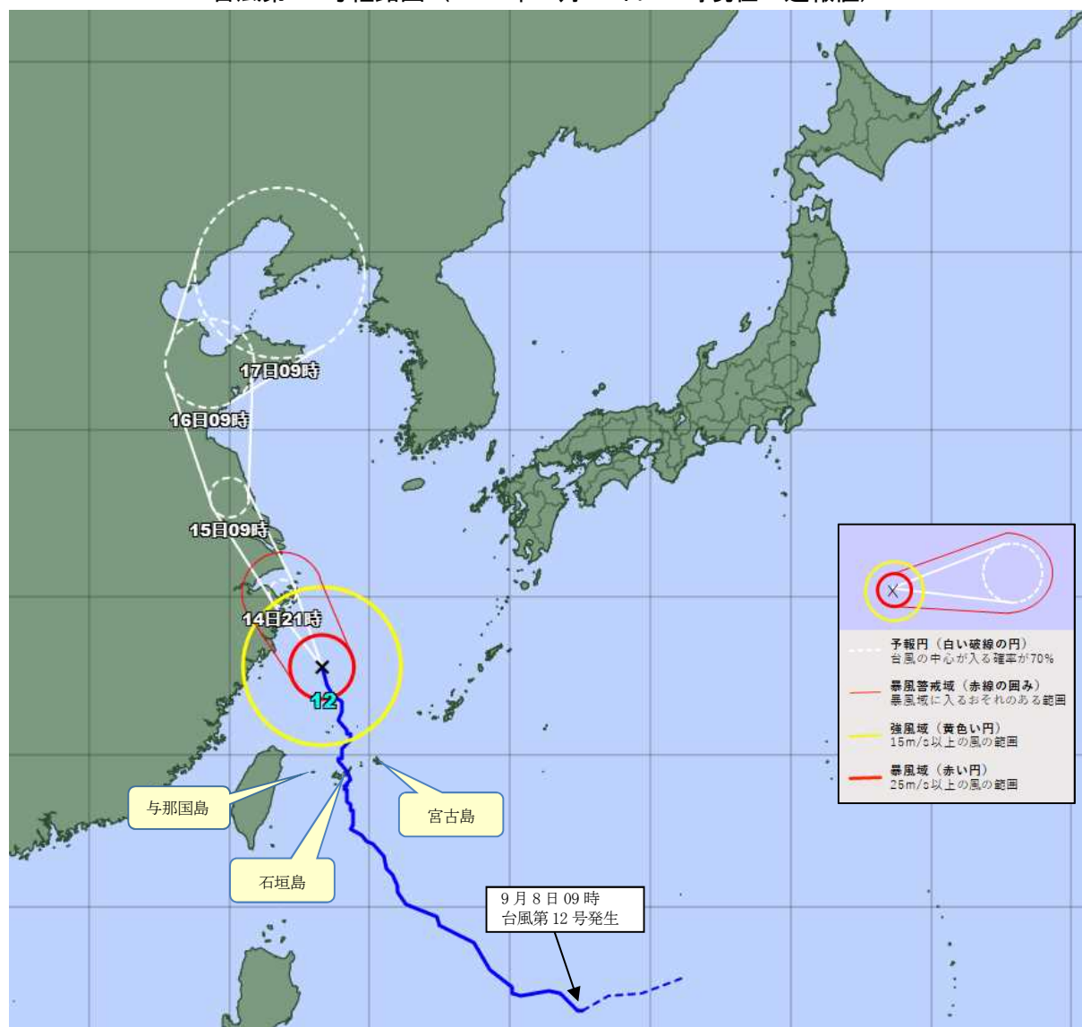
台風第12号経路図（2022年9月14日09時現在 速報値）
