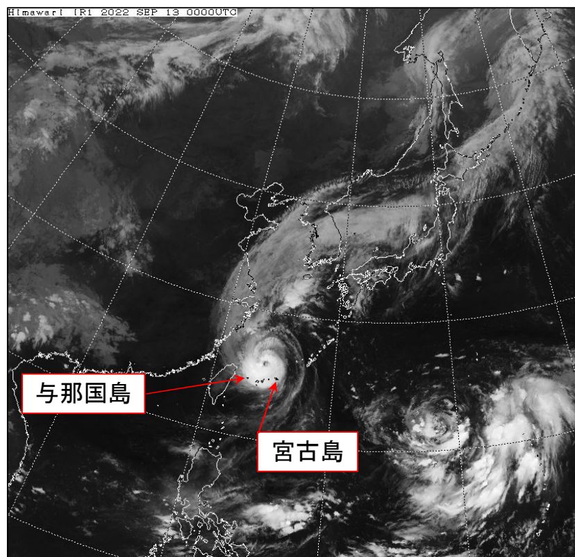
気象衛星画像（赤外） 2022年9月13日9時
