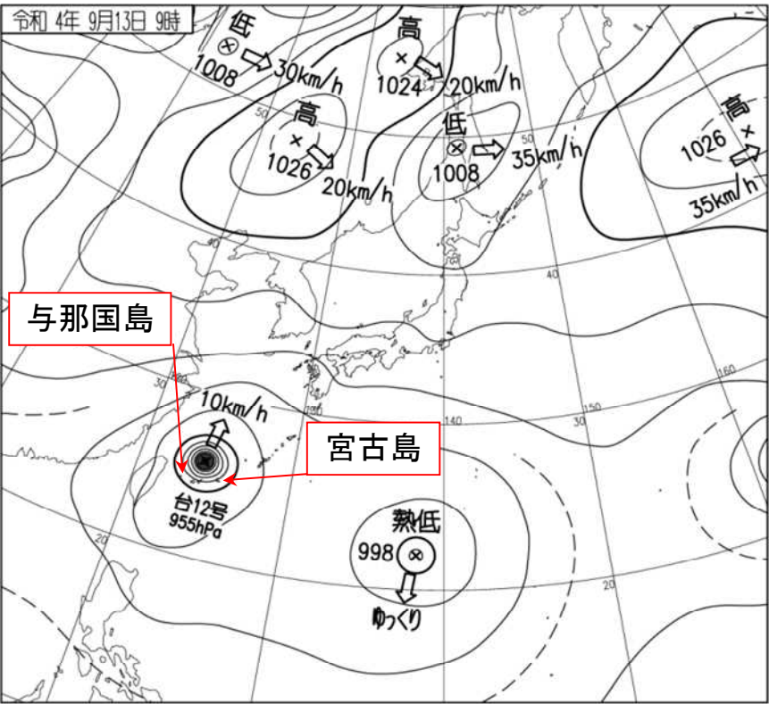
地上天気図 2022年9月13日9時
