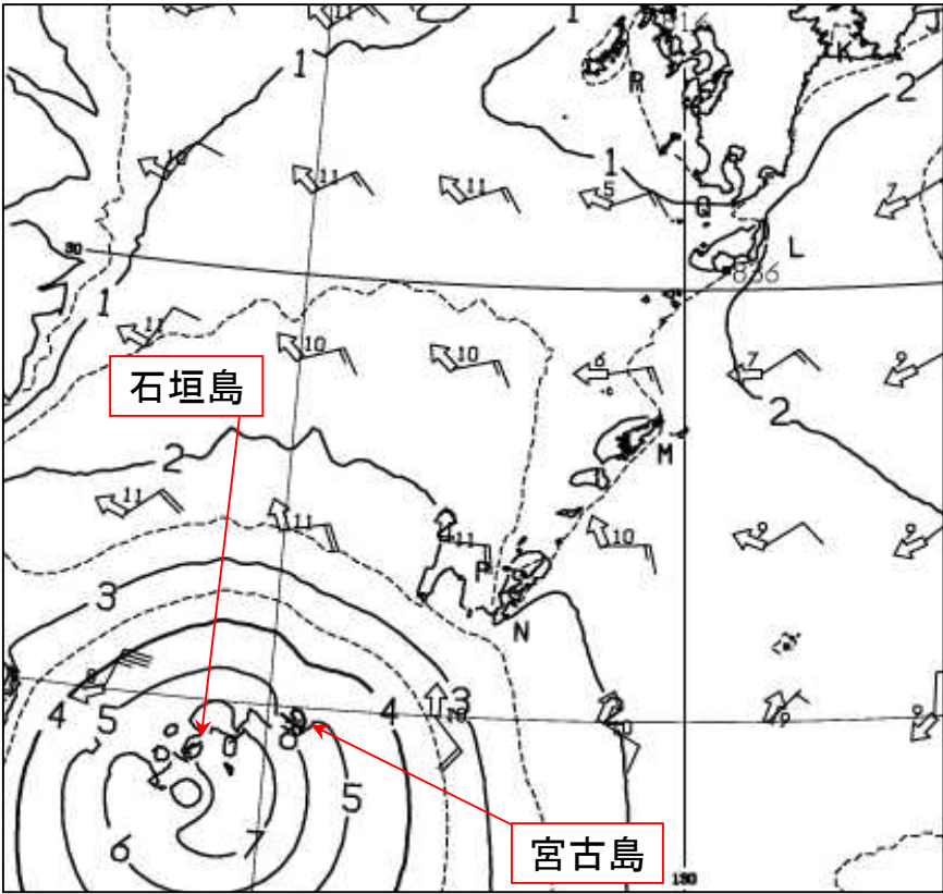
沿岸波浪実況図 2022年9月12日9時
