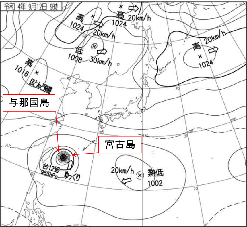
地上天気図 2022年9月12日9時
