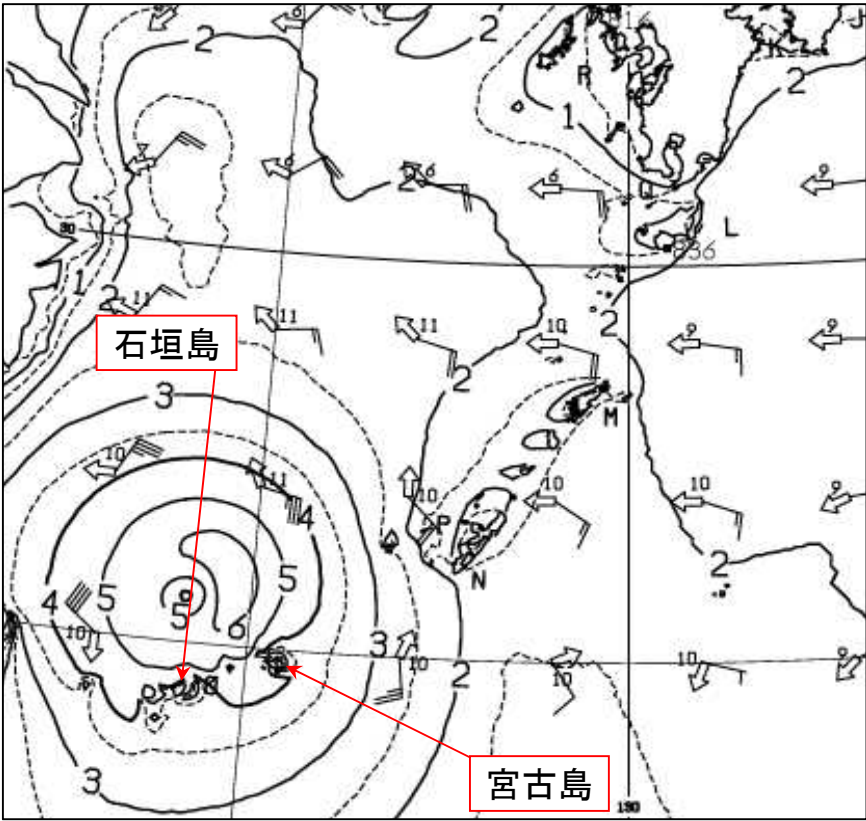
沿岸波浪実況図 2022年9月13日9時
