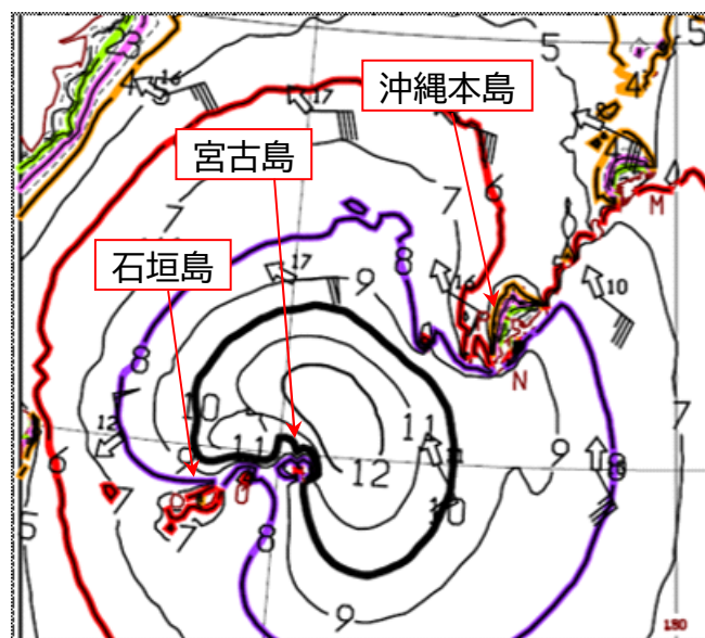
沿岸波浪実況図 2026年7月11日9時
