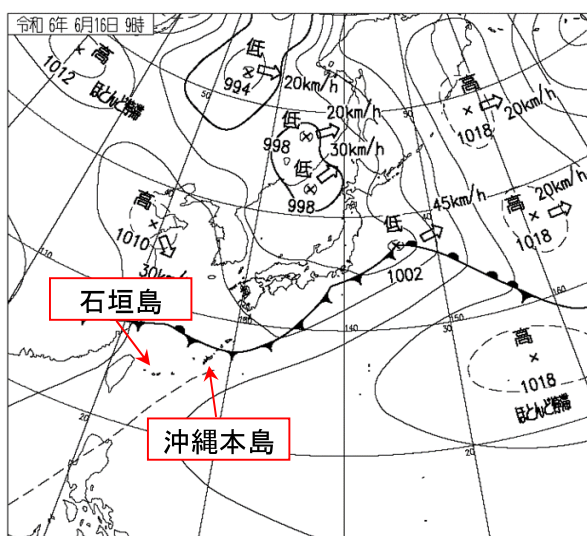
地上天気図 6月16日9時
