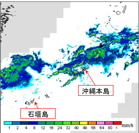
降水強度 6月14日9時
