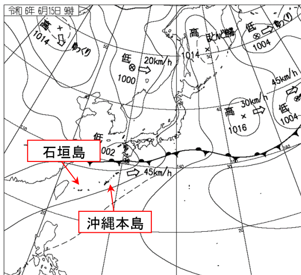
地上天気図 6月15日9時
