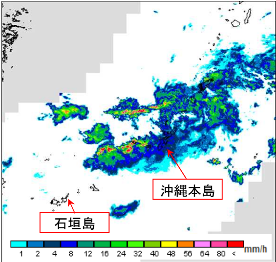
降水強度 6月11日9時
