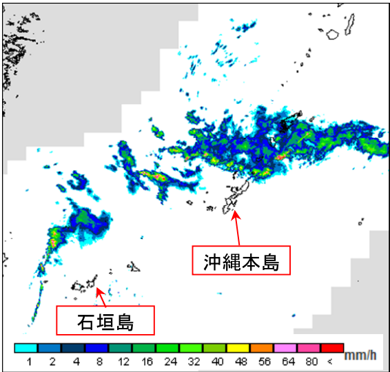
降水強度 6月19日9時
