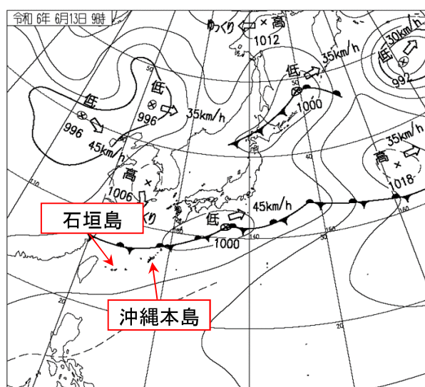
地上天気図 6月13日9時
