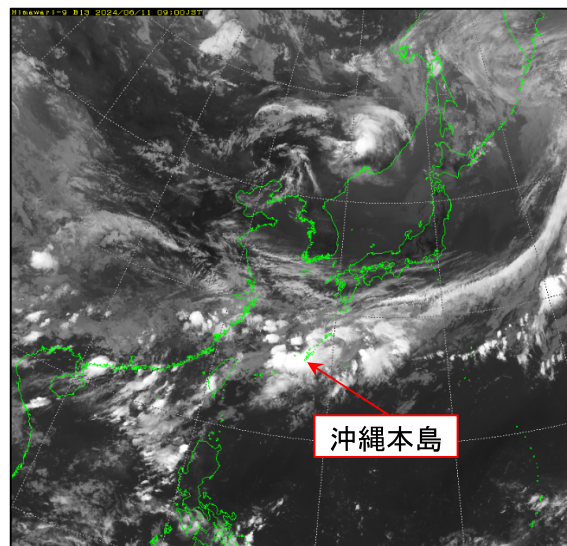
気象衛星画像(赤外) 6月11日9時
