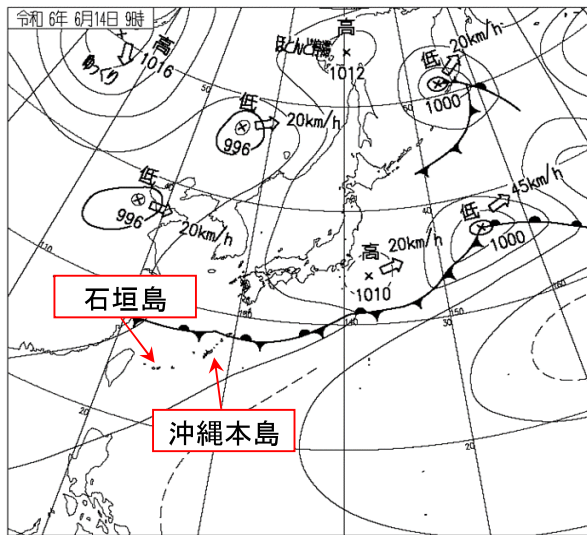
地上天気図 6月14日9時
