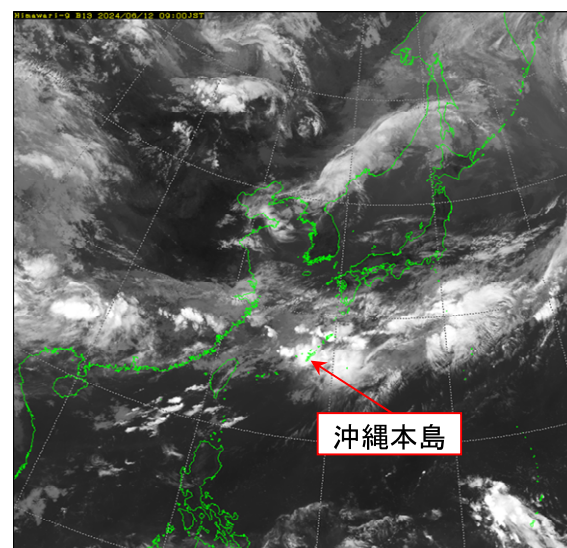
気象衛星画像(赤外) 6月12日9時
