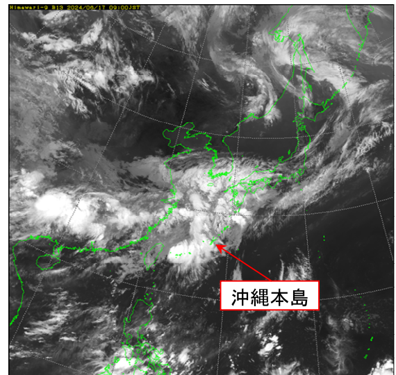
気象衛星画像(赤外) 6月17日9時
