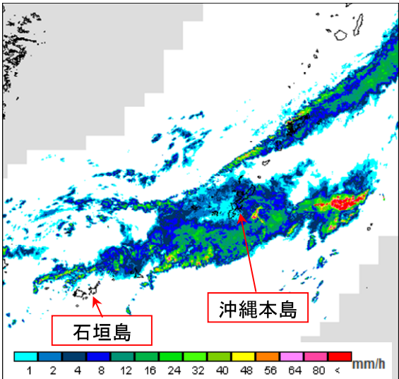
降水強度 6月18日9時
