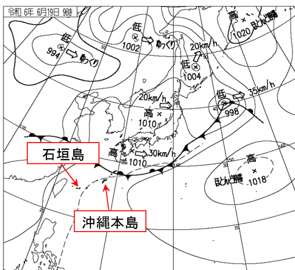
地上天気図 6月19日9時
