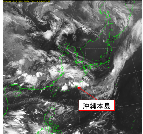
気象衛星画像(赤外) 6月19日9時
