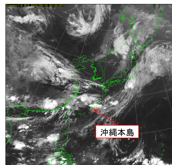
気象衛星画像(赤外) 6月16日9時
