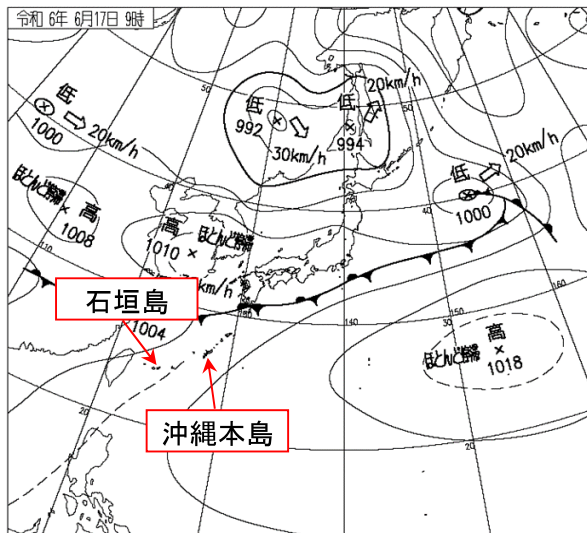
地上天気図 6月17日9時
