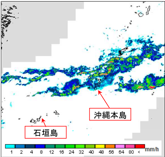
降水強度 6月13日9時
