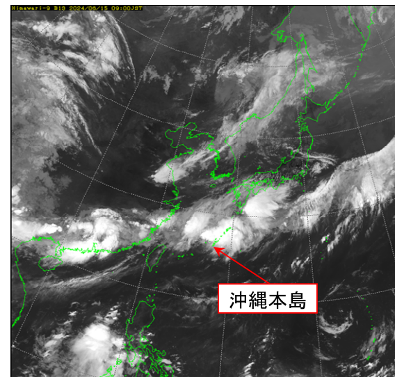
気象衛星画像(赤外) 6月15日9時
