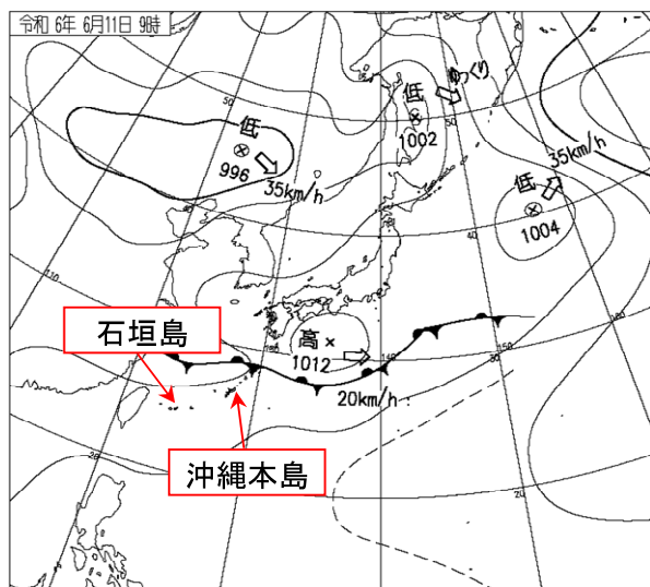
地上天気図 6月11日9時
