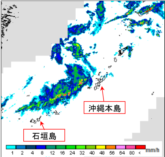
降水強度 6月17日9時
