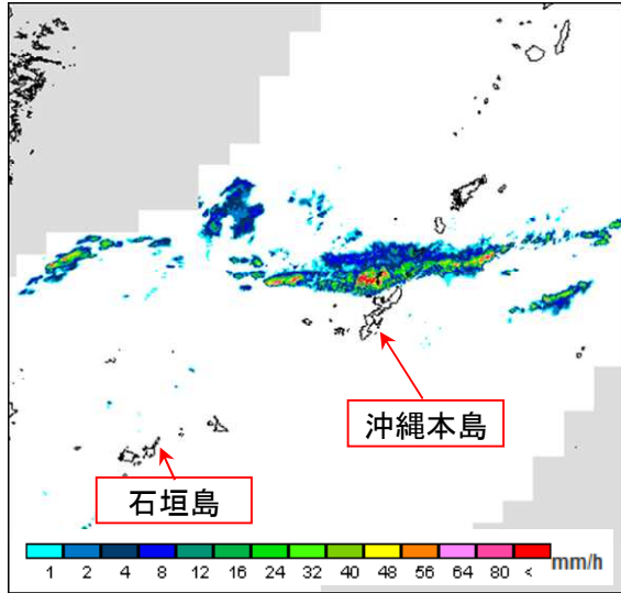
降水強度 6月16日9時
