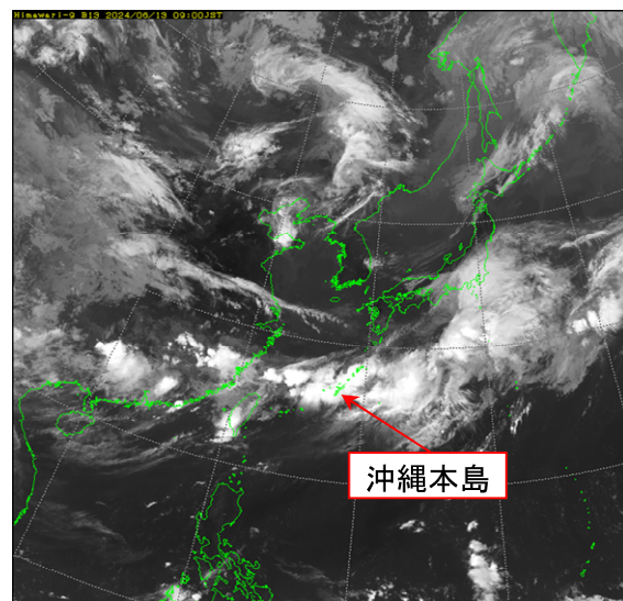
気象衛星画像(赤外) 6月13日9時
