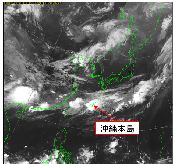
気象衛星画像(赤外) 6月14日9時
