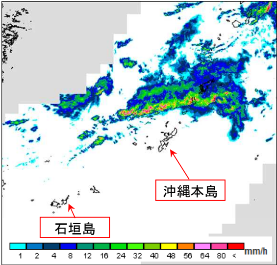
降水強度 6月15日9時
