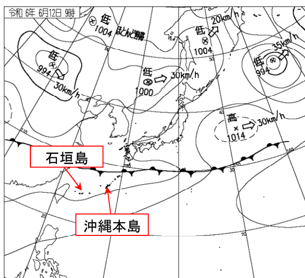
地上天気図 6月12日9時
