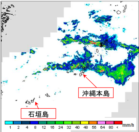
降水強度 6月12日9時
