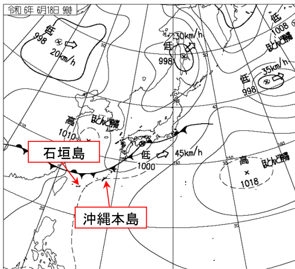
地上天気図 6月18日9時
