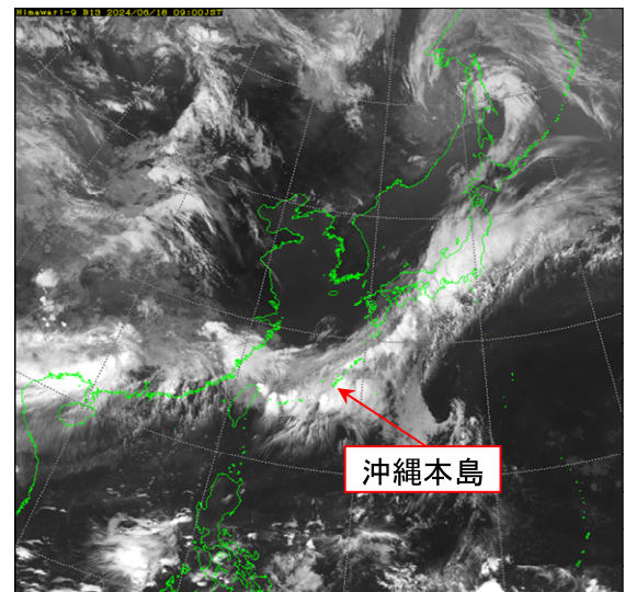
気象衛星画像(赤外) 6月18日9時
