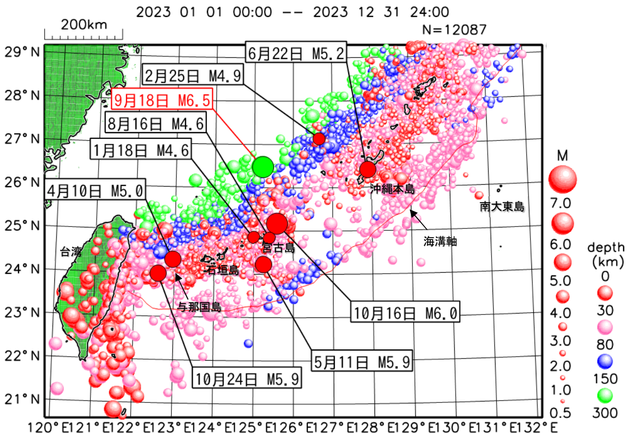
第1図 沖縄地方とその周辺の震央分布図（2023年1月1日～12月31日）
