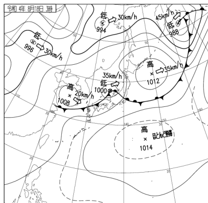
地上天気図
