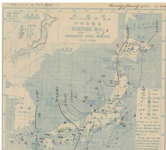
明治25年1月7日6時の天気図 最低気温 -27.2℃
