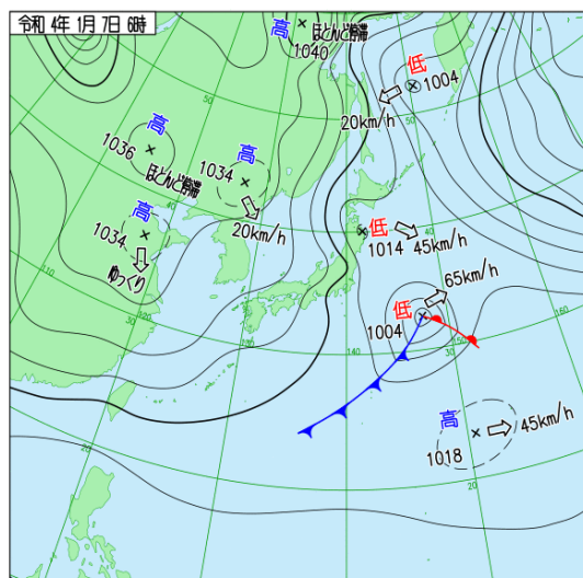
令和4年1月7日6時の天気図 最低気温 -12.8℃
