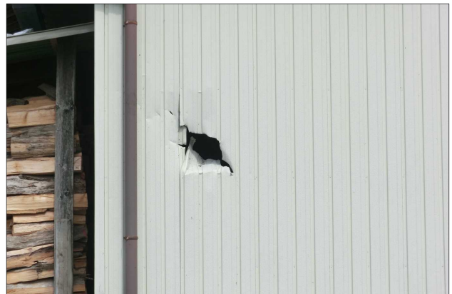
⑥ 飛散したスレートにより損傷した トタンの壁 (西方向から撮影)
