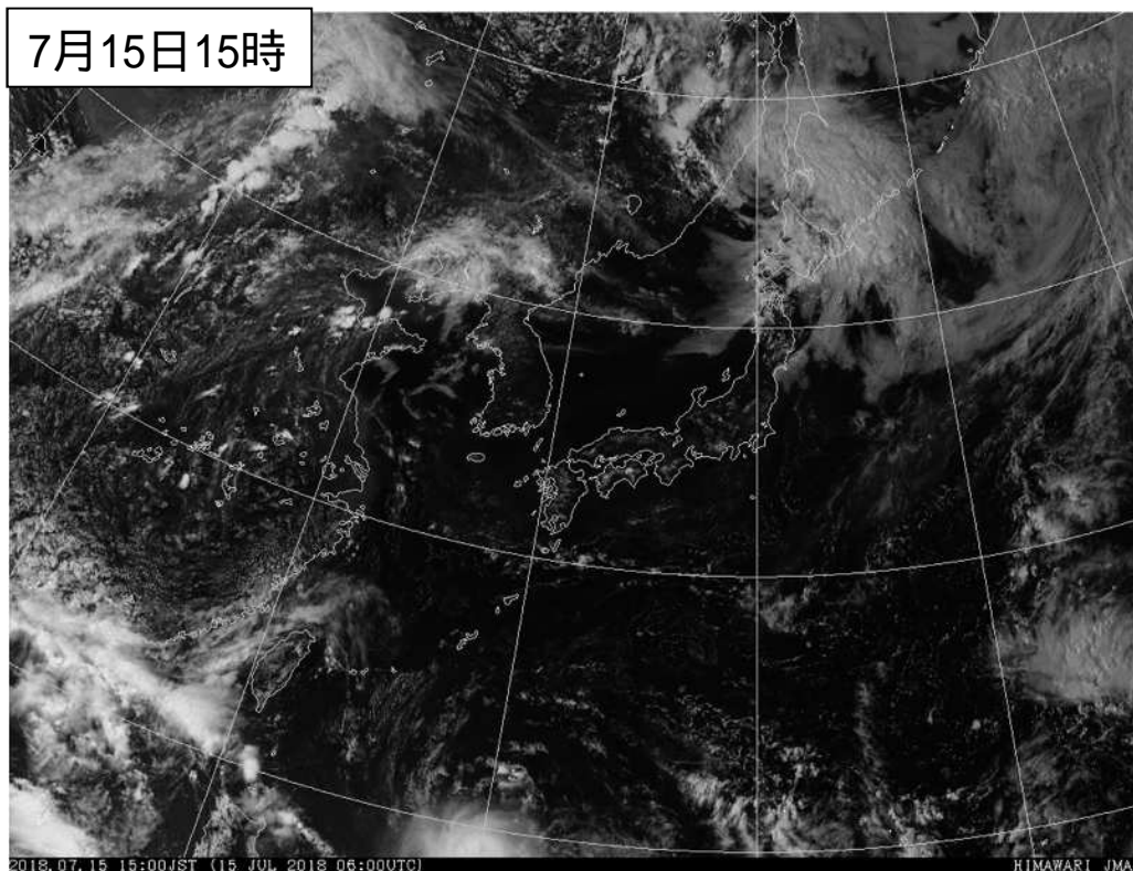
地上天気図および気象衛星「ひまわり8号」可視画像
