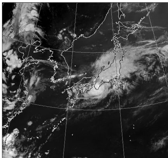
気象衛星赤外面像(7月4日17時)
