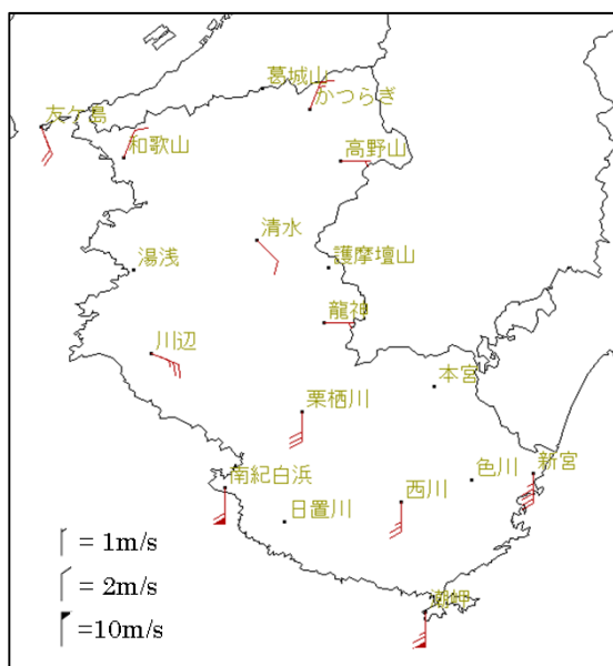
アメダス地点における前10分間平均風向風速分布図 (7月4日16時30分)
