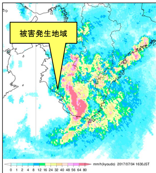
気象レーダー画像(降水強度) (7月4日16時30分)
