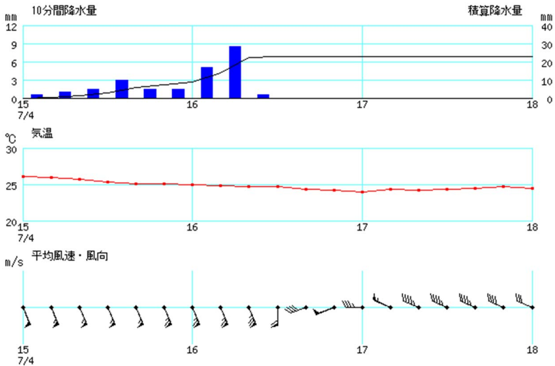
アメダス南紀白浜 時系列グラフ(7月4日15時~18時)
