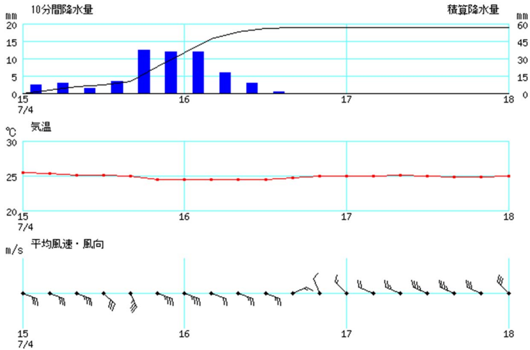
アメダス川辺 時系列グラフ(7月4日15時~18時)
