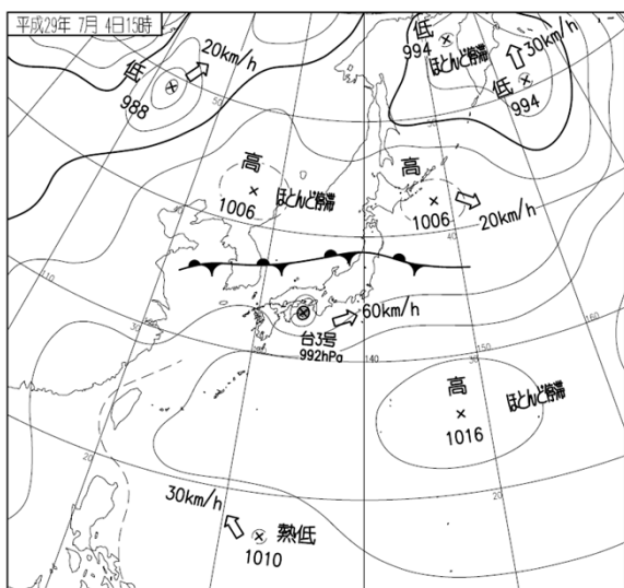
地上天気図(7月4日15時)
