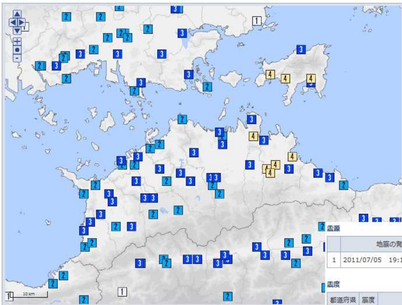
震度分布図
