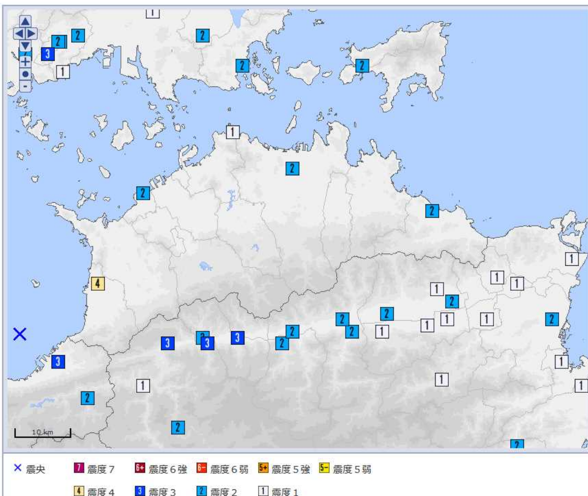
震度分布図
