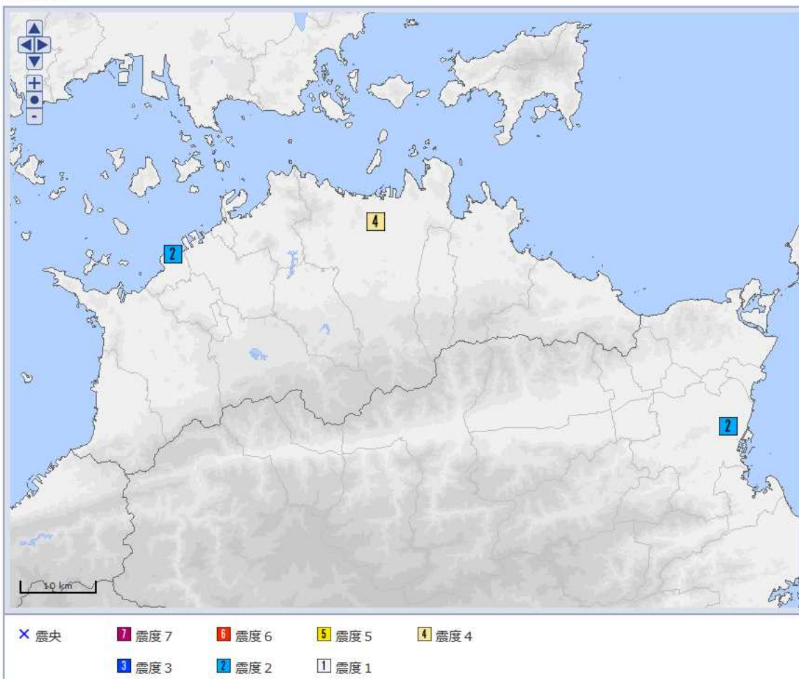
震度分布図
