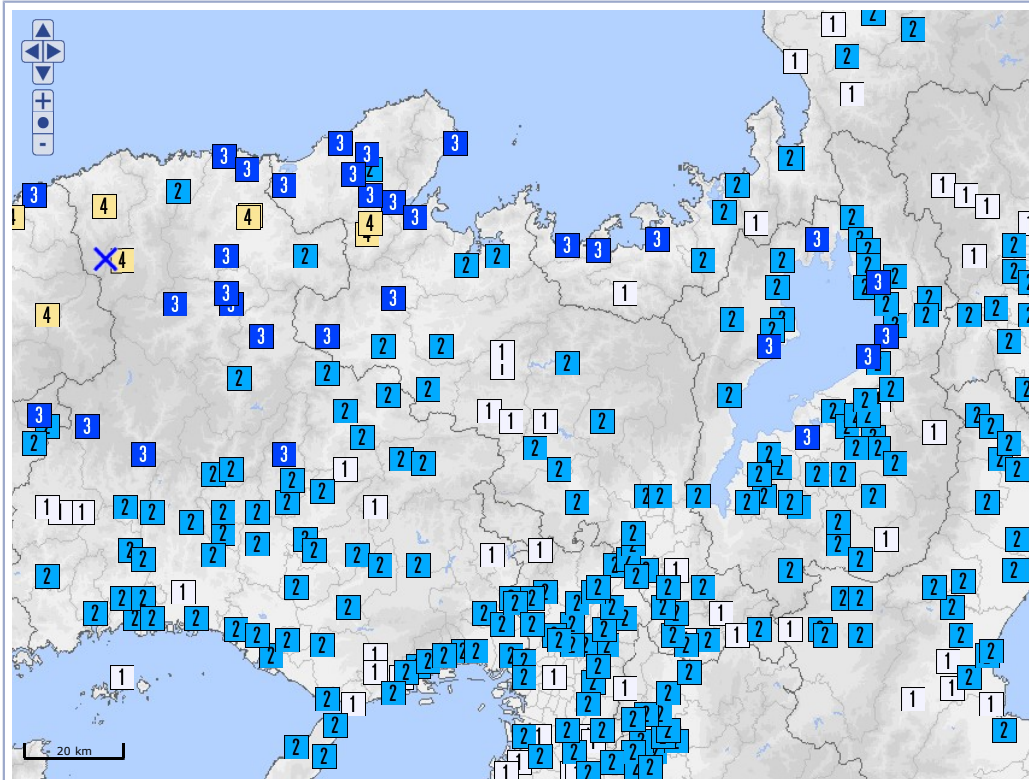
震度分布図
