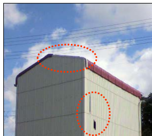
⑥屋根および壁の一部が破損した倉庫 （南西から撮影）
