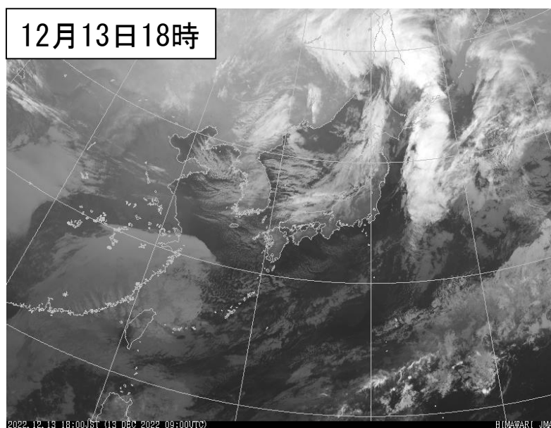
地上天気図及び気象衛星赤外画像
