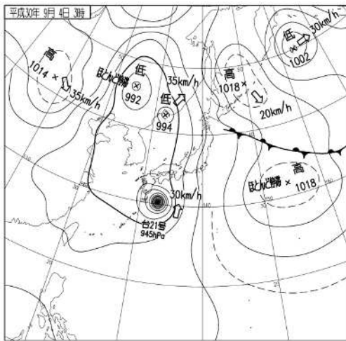
地上天気図 ( 9 月 4 日 03 時 )
