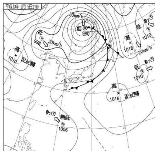
地上天気図 (9月5日 21時)
