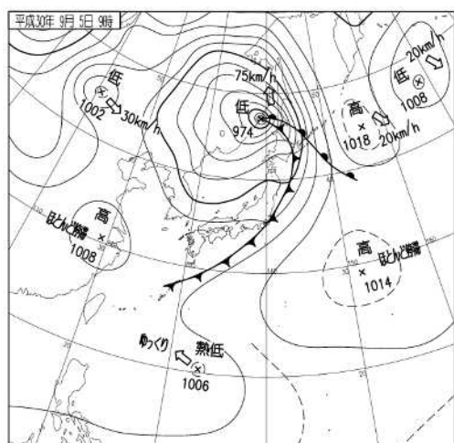
地上天気図 (9月5日 09時)
