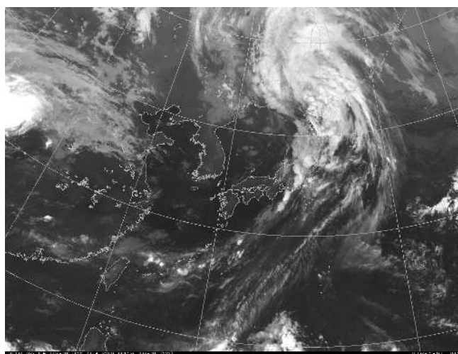
気象衛星赤外画像 (9月5日 03時)
