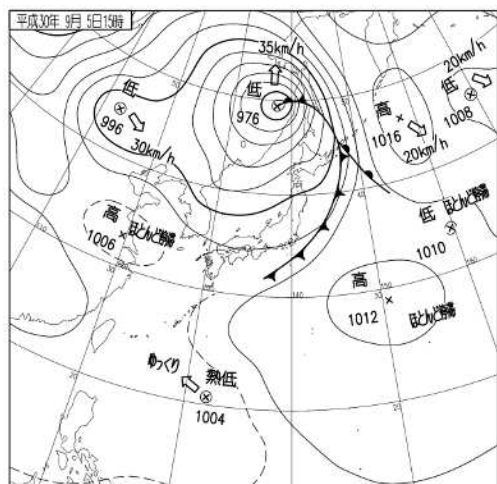
地上天気図 (9月5日 15時)
