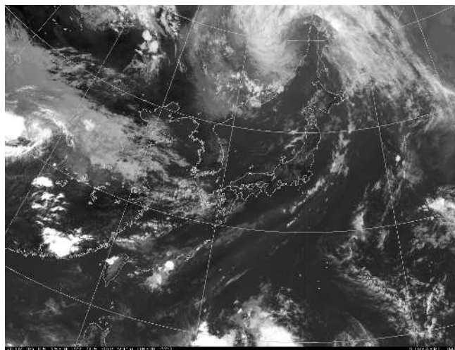
気象衛星赤外画像 (9月5日 15時)
